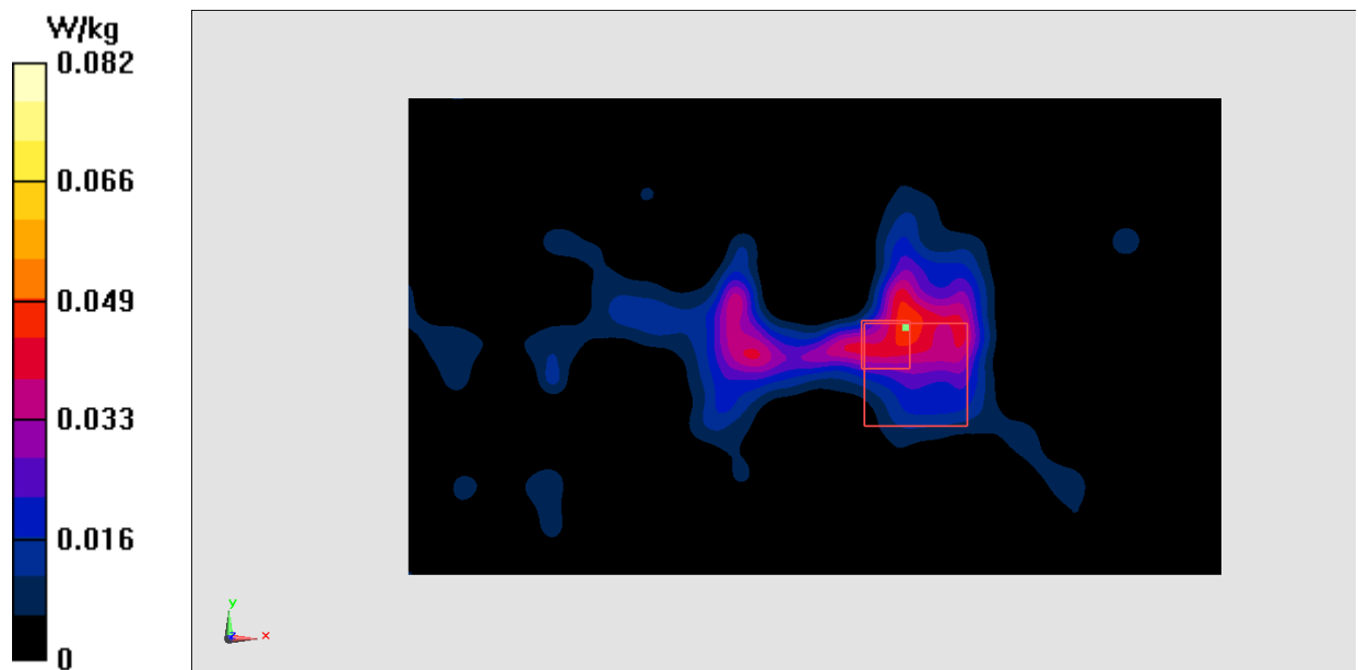
Fig.14 5GHz
