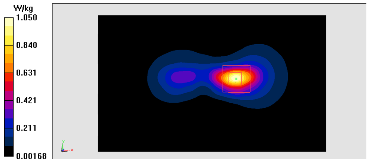
Fig.10 LTE Band7
