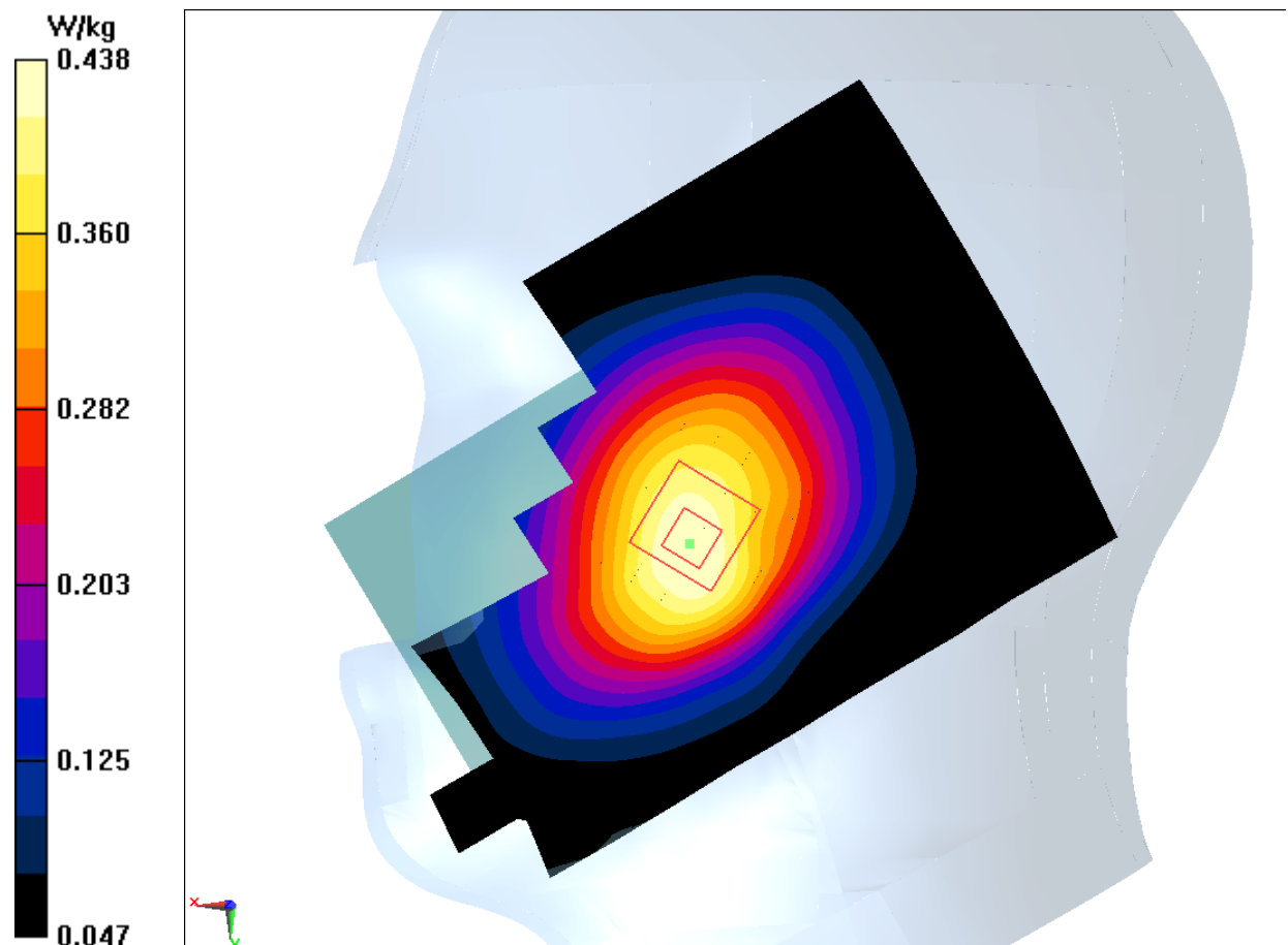
Fig.5 WCDMA 850
