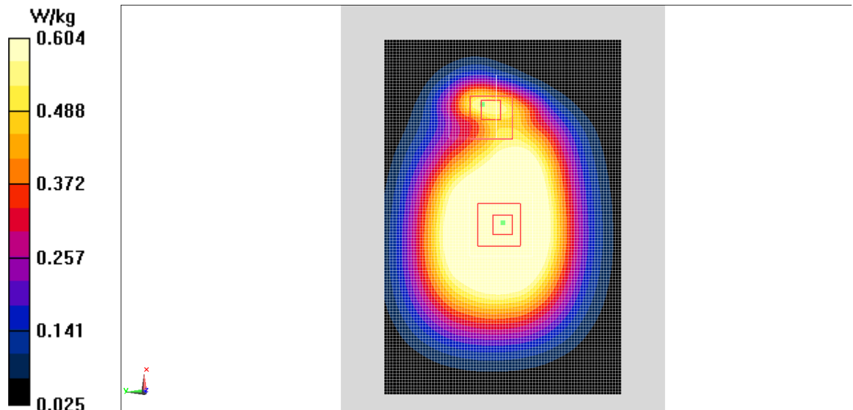
Fig.6 WCDMA 850
