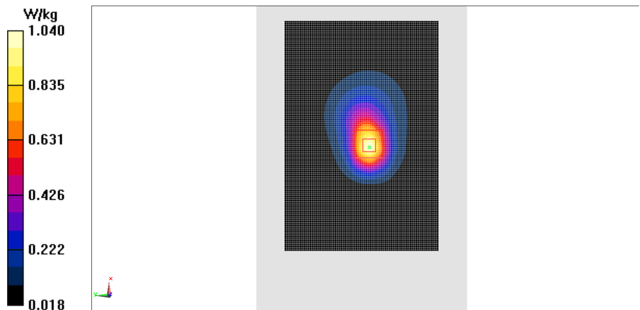
Fig.8 WCDMA1900
