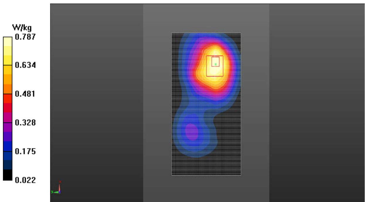
Fig.8 WCDMA1900 CH9400
