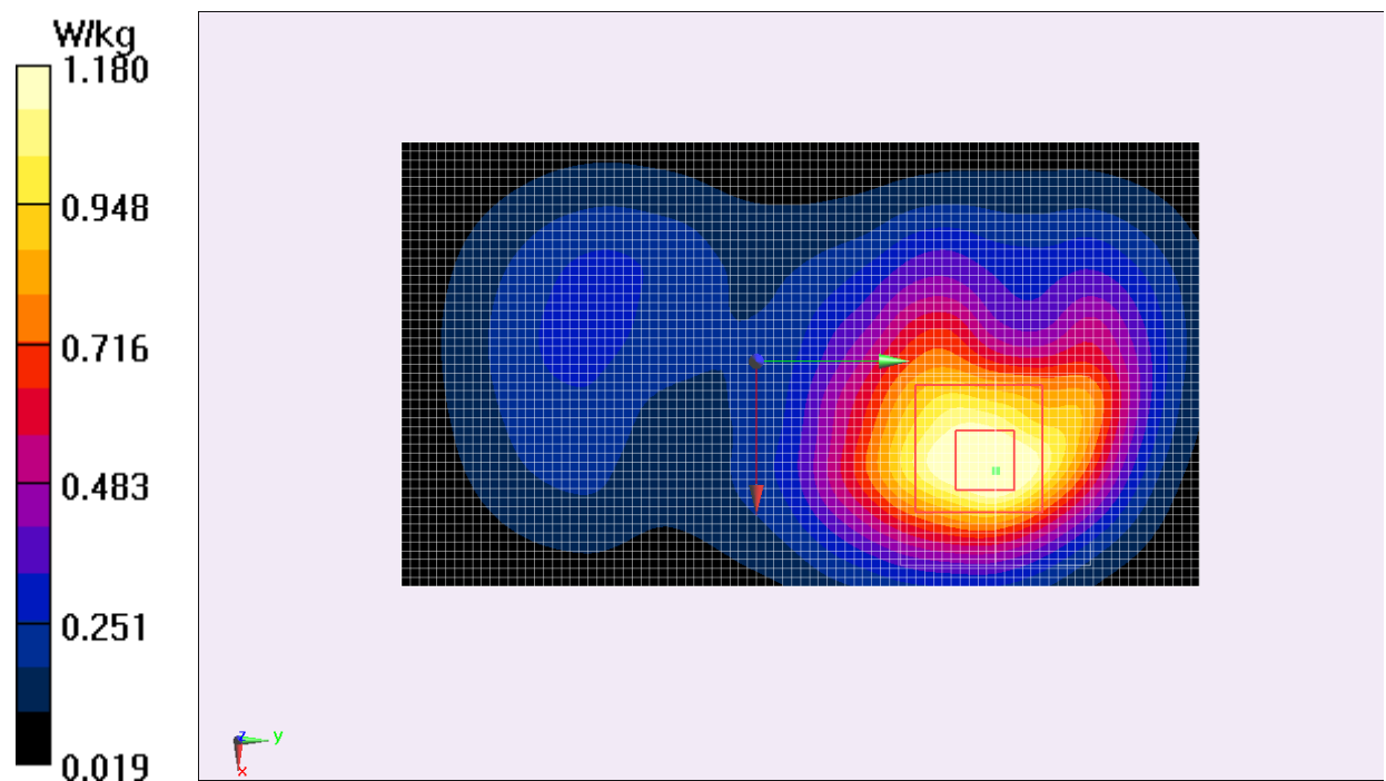
Fig.8 WCDMA1900 CH9538
