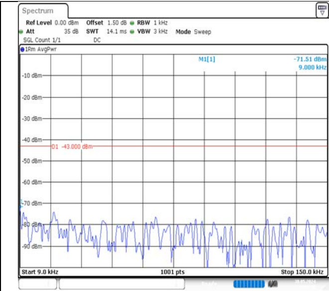
Band4-20MHz-QPSK-20175-1RB#0-0.009~0.15-PASS
