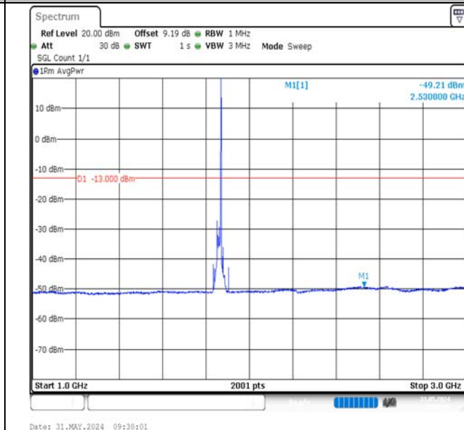
Band2-20MHz-QPSK-18700-1RB#99-1000~3000-PASS
