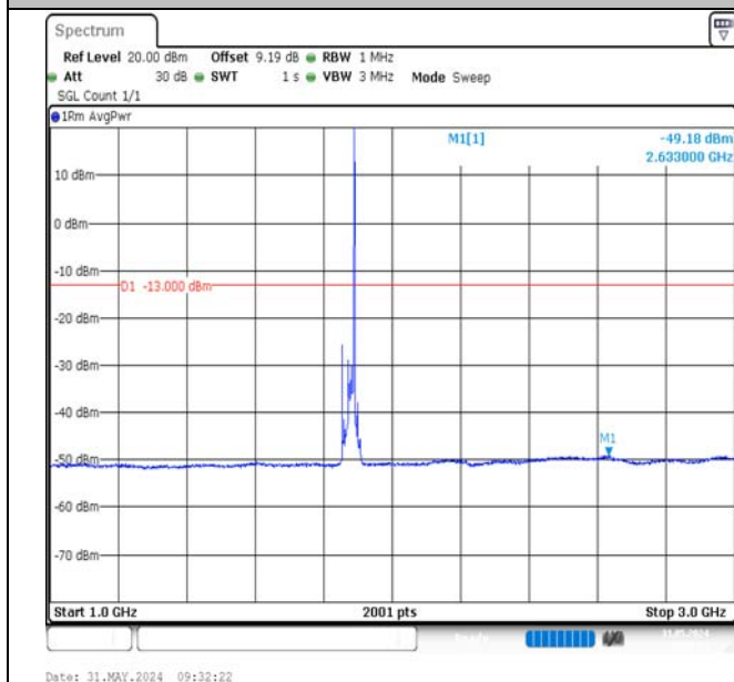
Band2-20MHz-QPSK-18900-1RB#99-1000~3000-PASS
