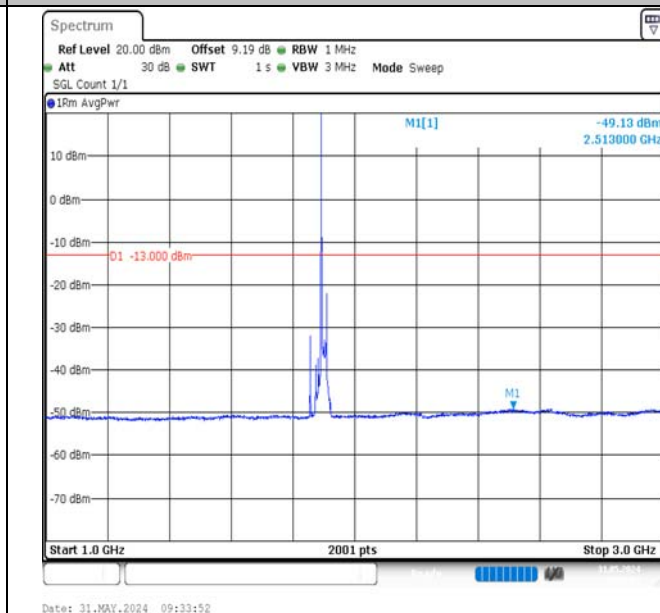
Band2-20MHz-QPSK-19100-1RB#0-1000~3000-PASS
