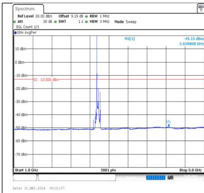
Band2-20MHz-QPSK-18900-1RB#0-1000~3000-PASS
