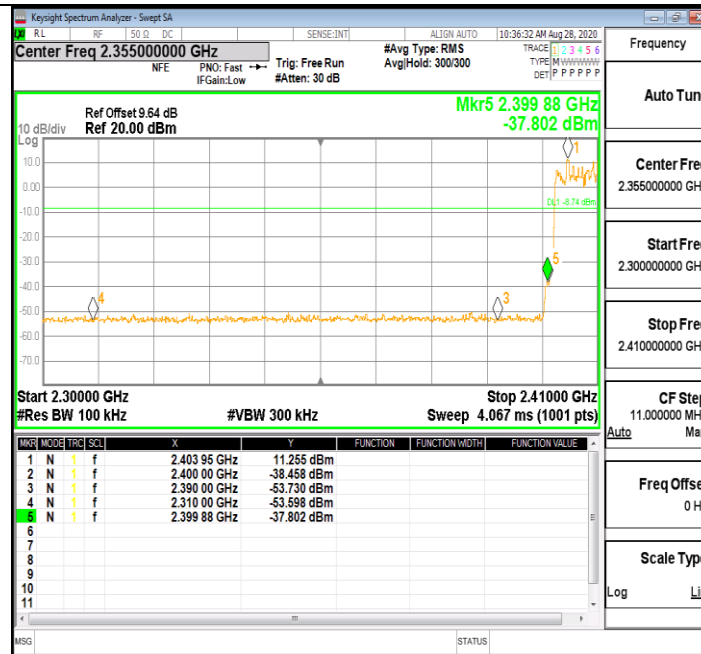
3DH5_Ant1_Low_Hop_2402
