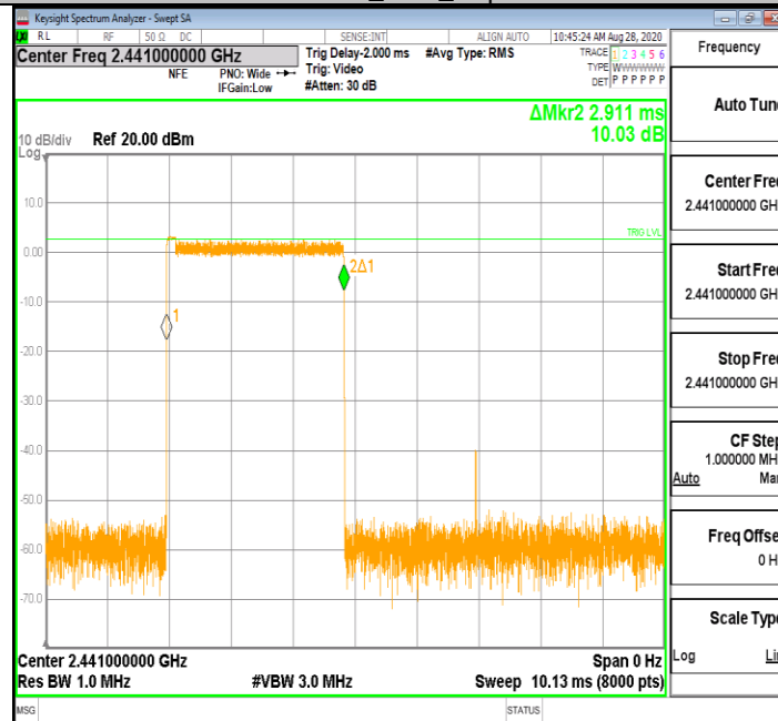
3DH5_Ant1_Hop
