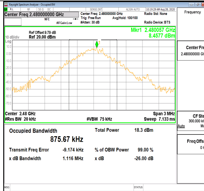
DH5_Ant1_2480
