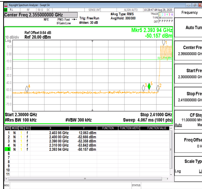
DH5_Ant1_Low_Hop_2402
