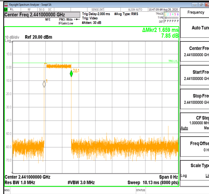
3DH3_Ant1_Hop
