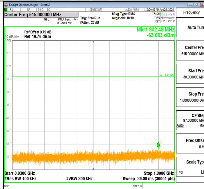
DH5_Ant1_2480_30~1000
