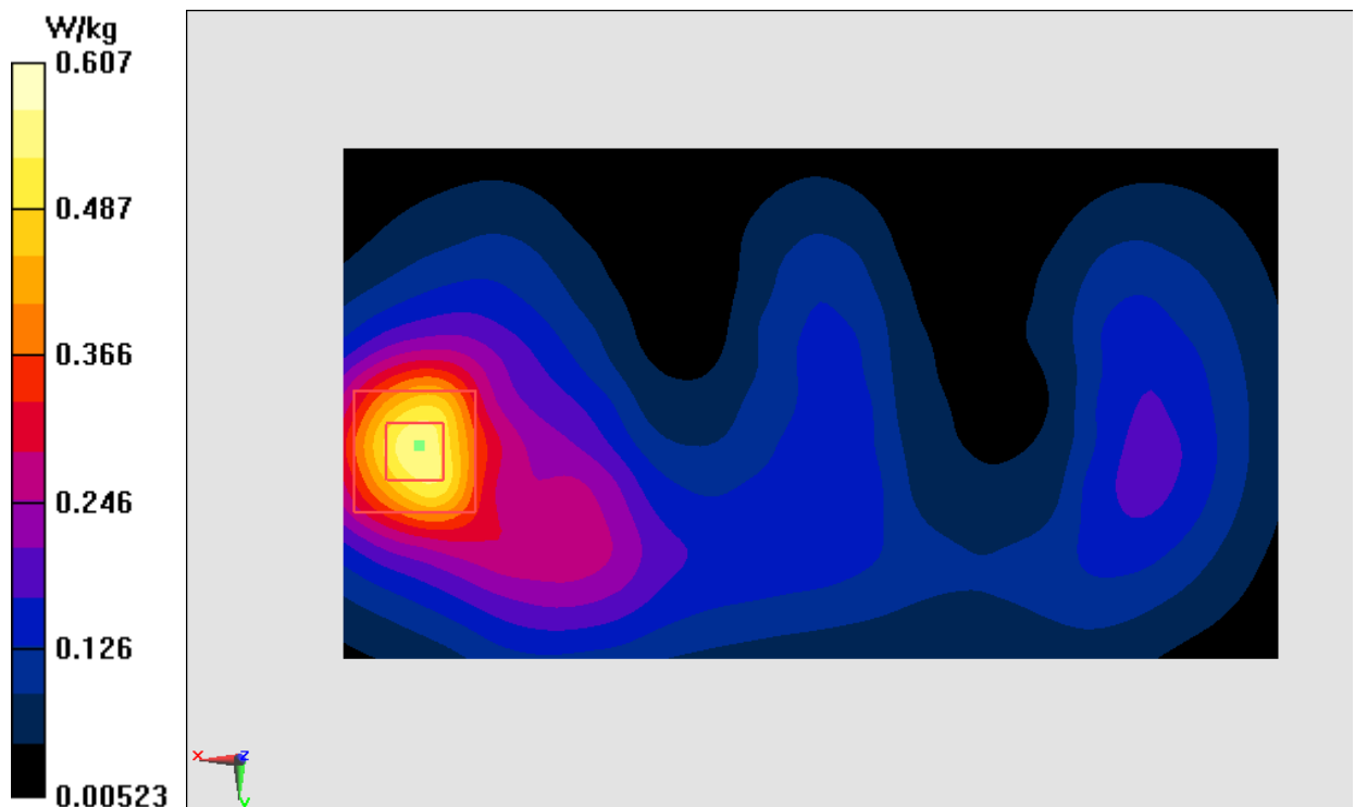
Fig.20 LTE Band7
