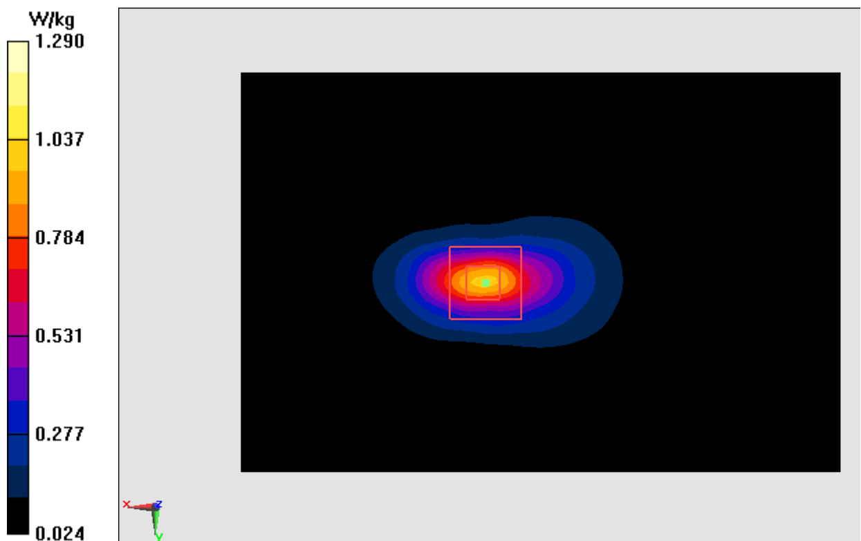
Fig.24 WCDMA1700
