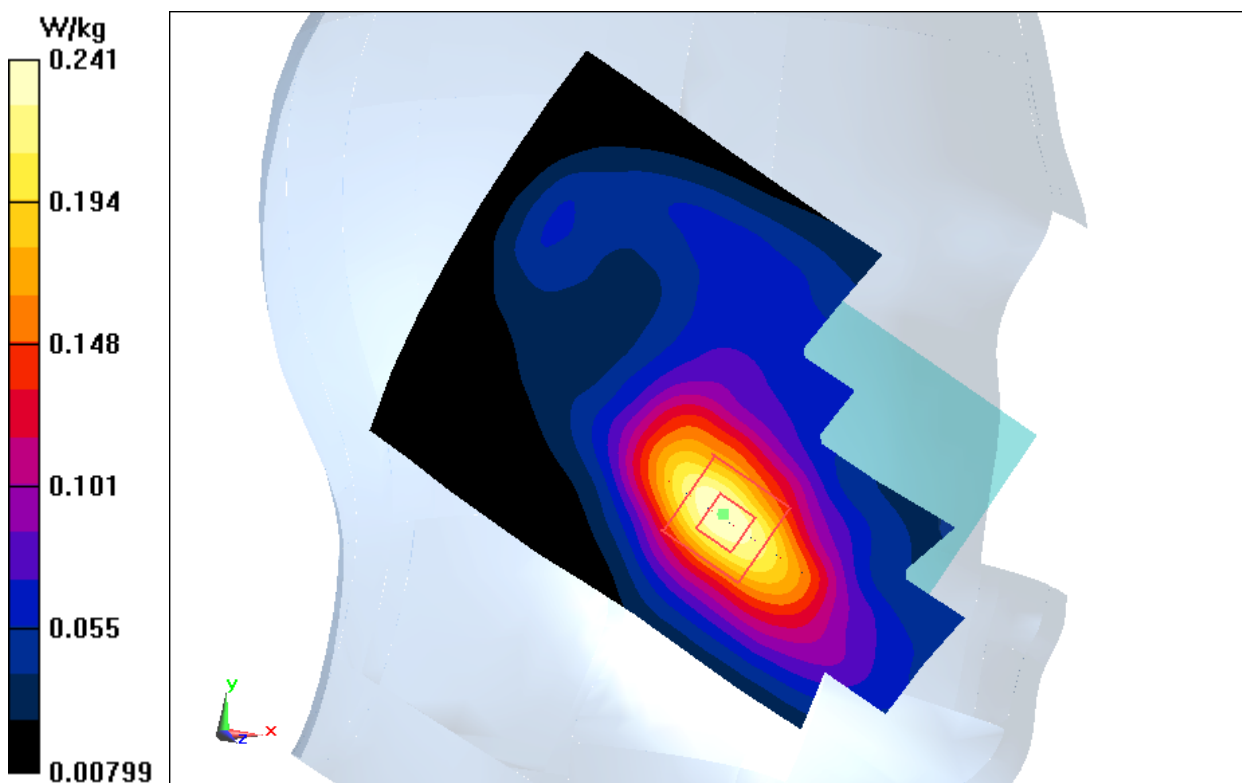
Fig.23 WCDMA1700
