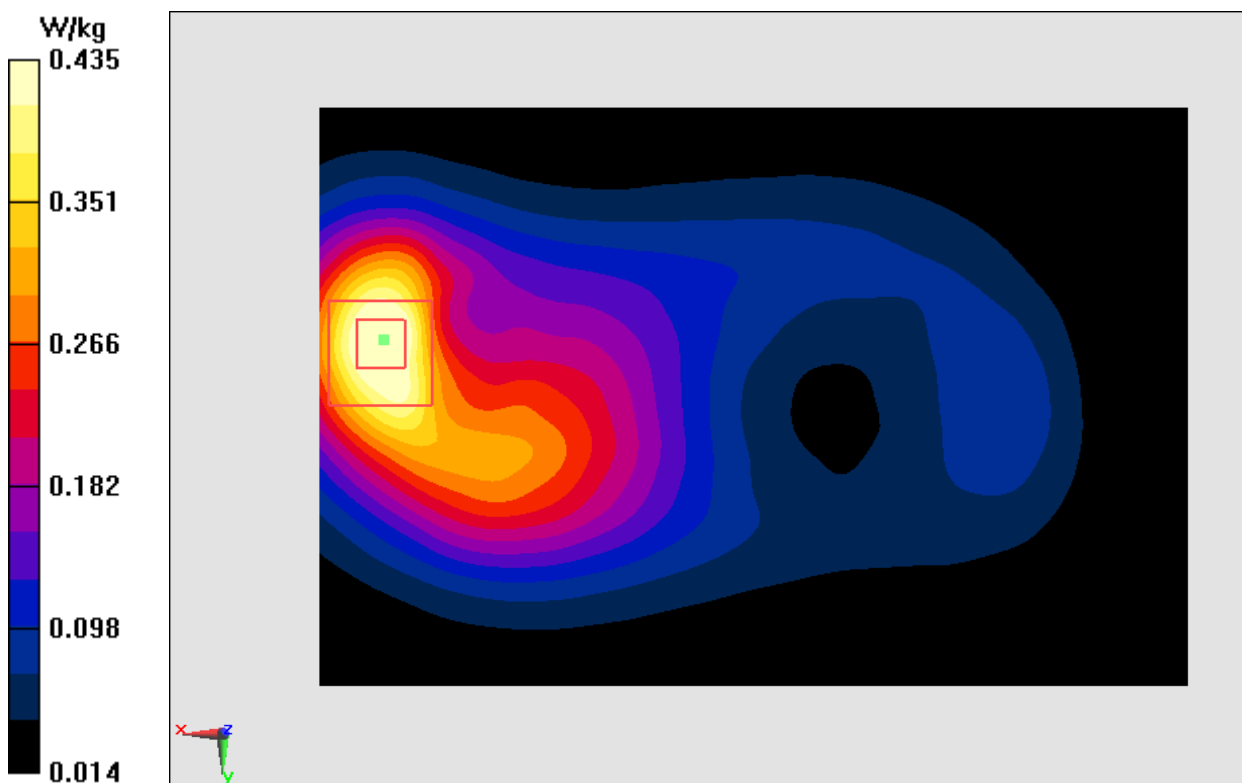
Fig.25 WCDMA1700
