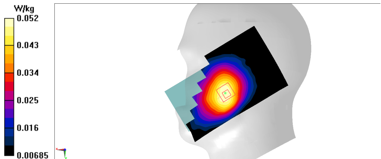
Fig.5 WCDMA 850
