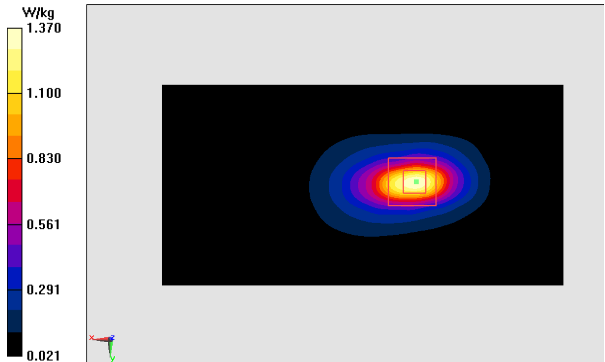
Fig.10 WCDMA1900
