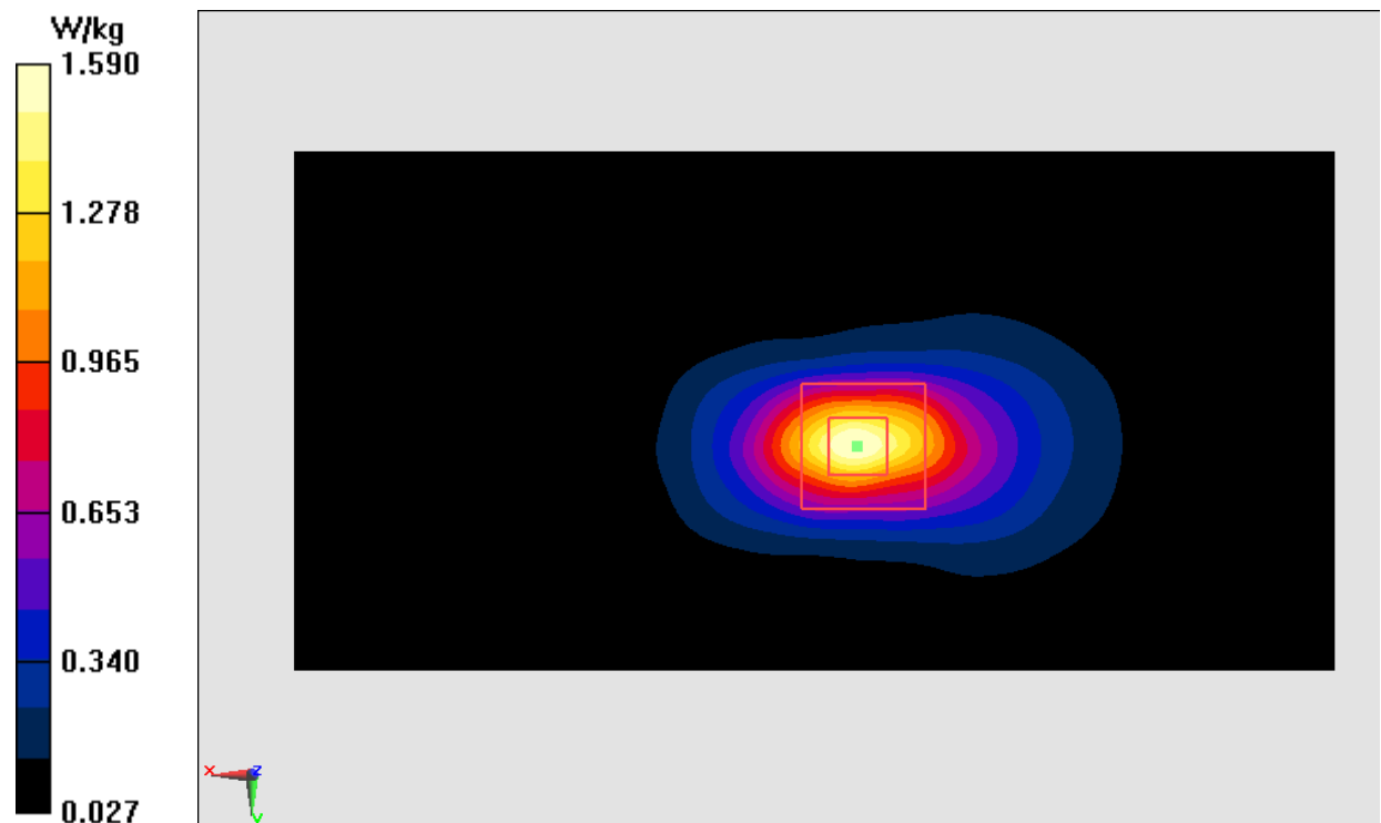
Fig.8 WCDMA1700
