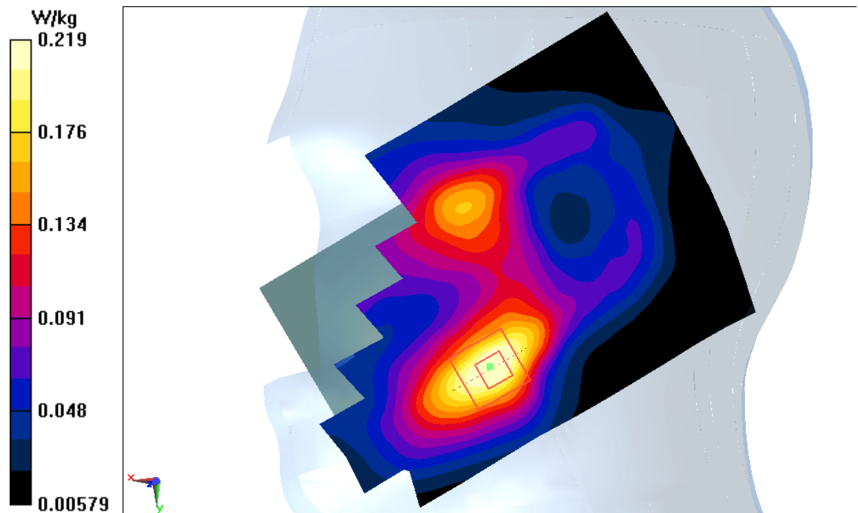
Fig.7 WCDMA1700
