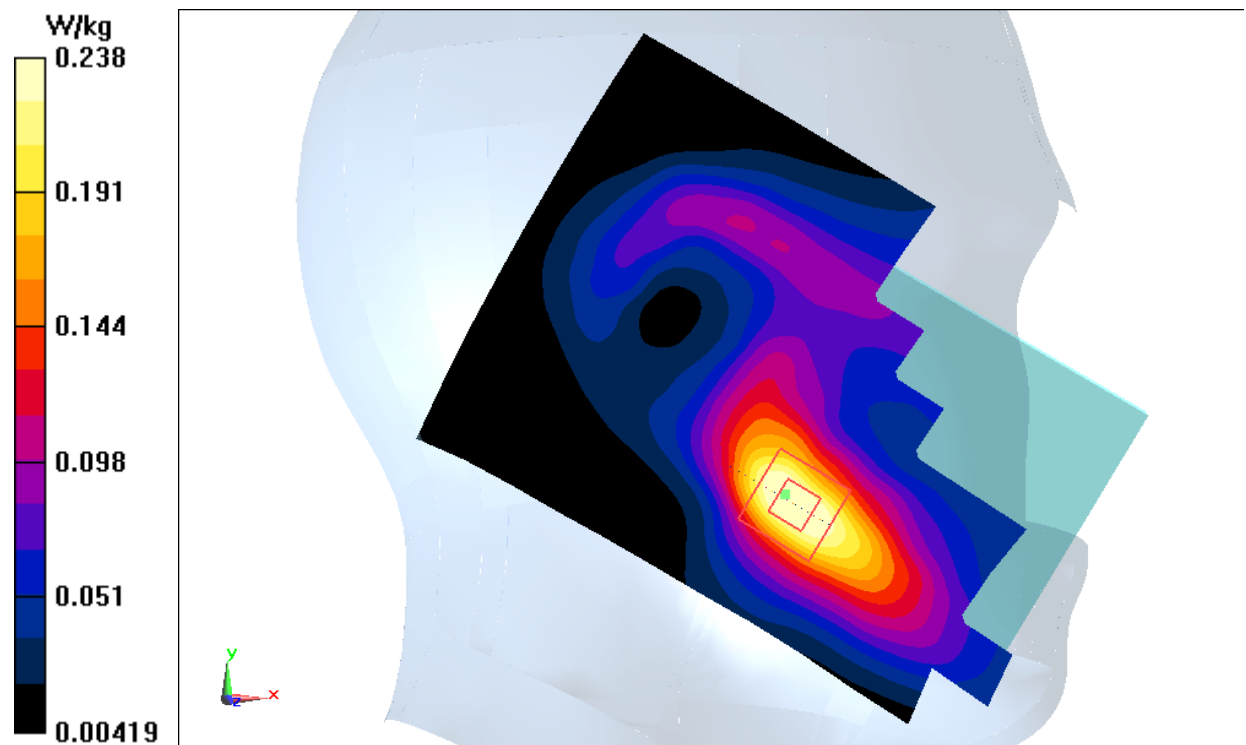
Fig.9 WCDMA1900
