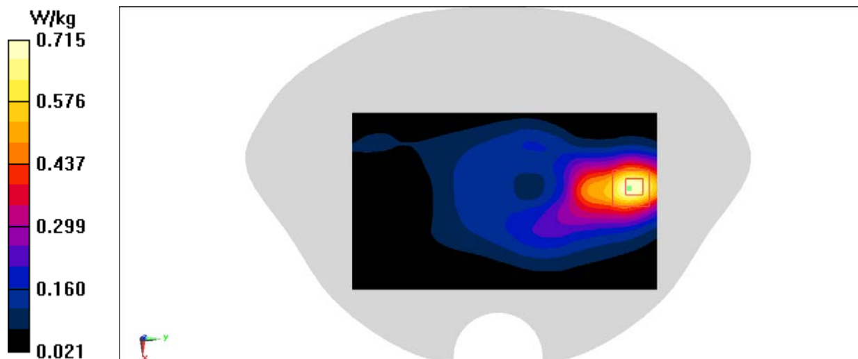
Fig.32 CDMA BC1
