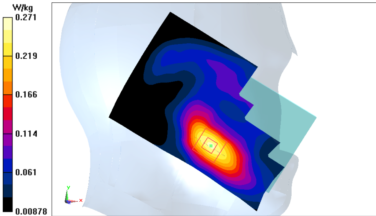
Fig.30 CDMA BC1
