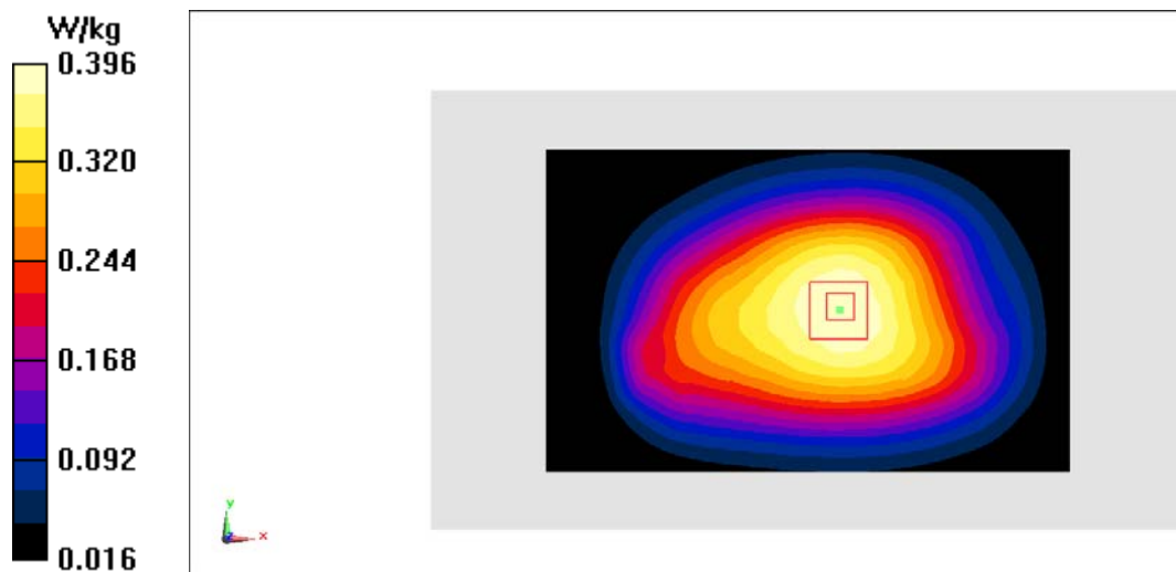
Fig.27 LTE Band13
