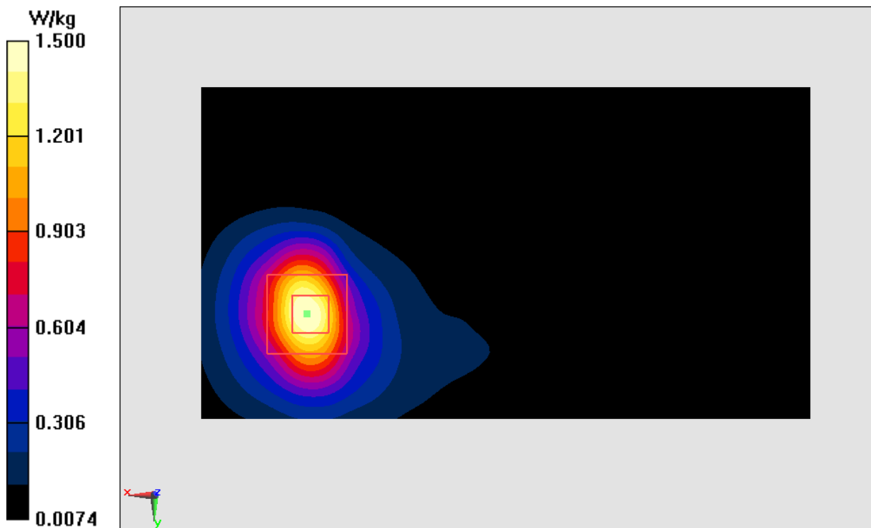
Fig.23 LTE Band7
