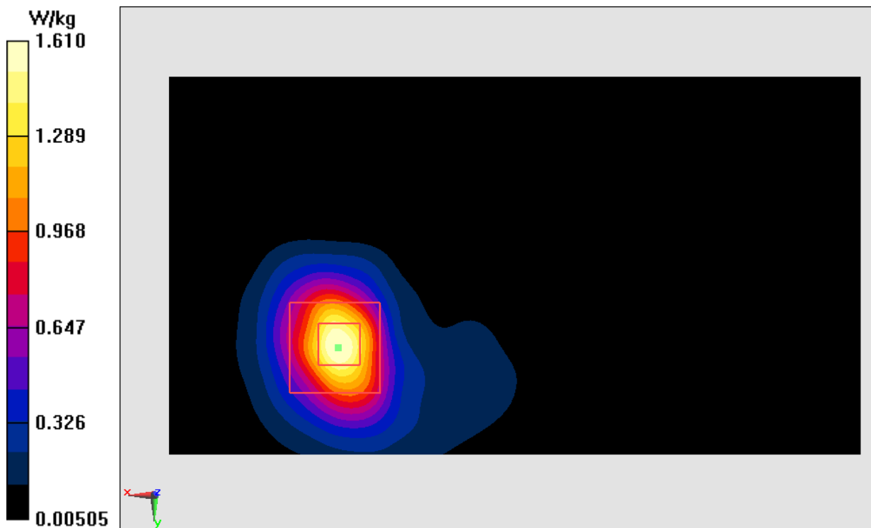
Fig.22 LTE Band7
