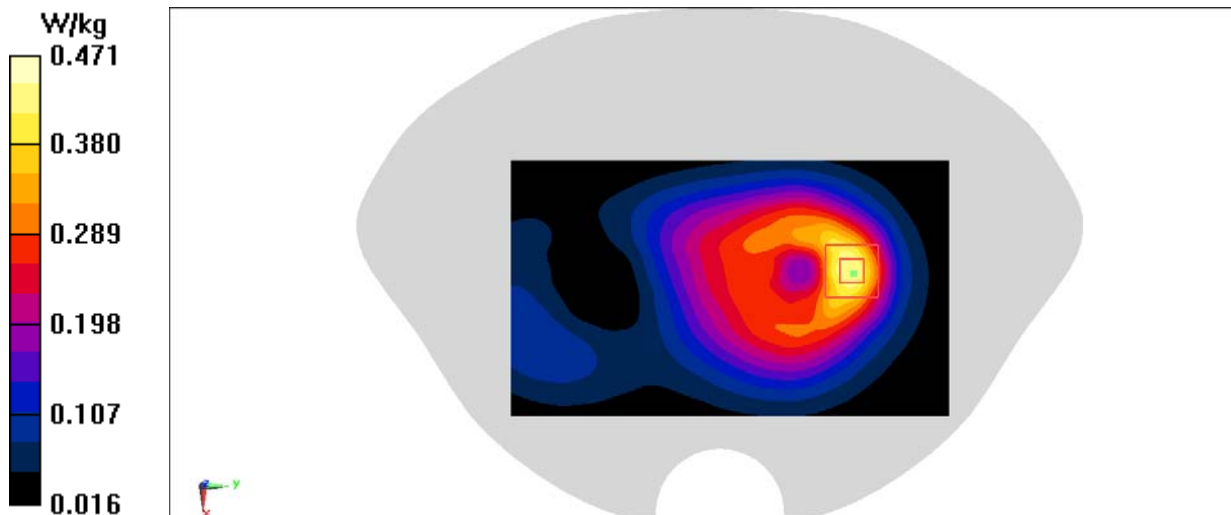
Fig.18 LTE Band4
