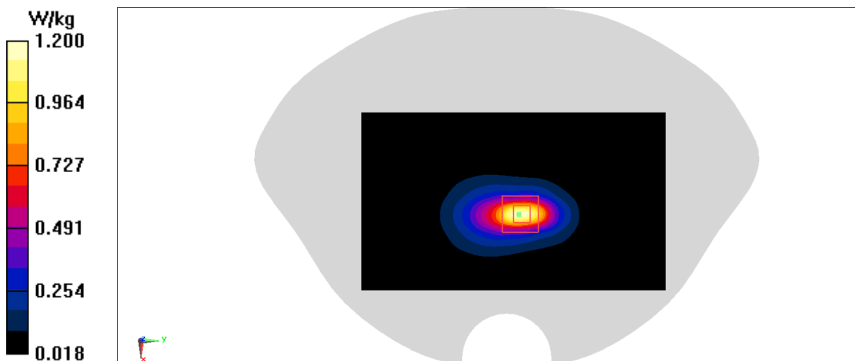
Fig.31 CDMA BC1
