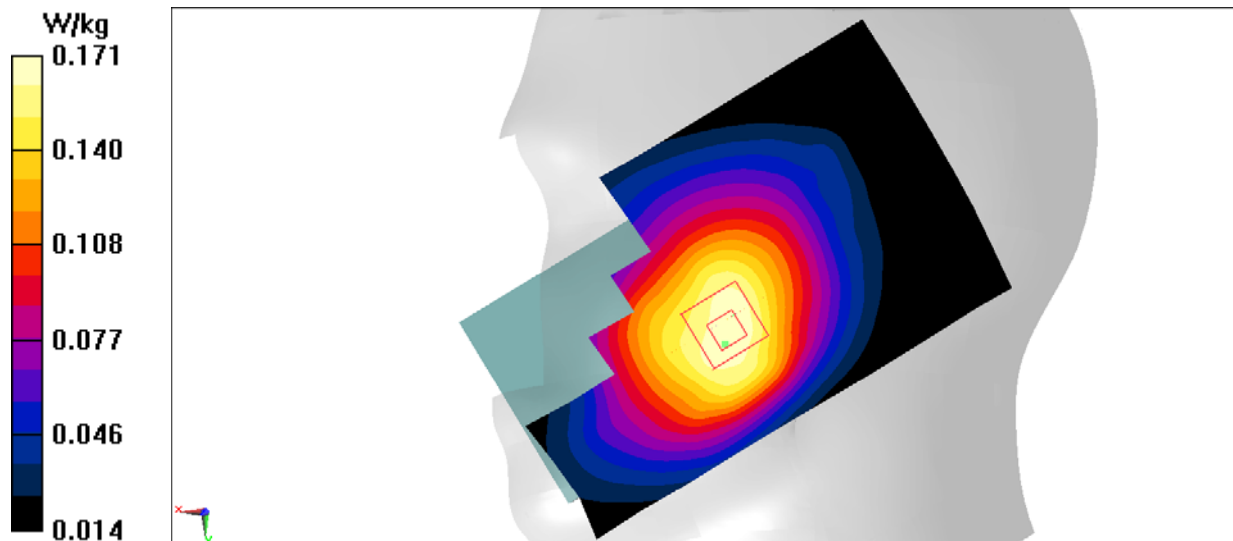
Fig.26 LTE Band13
