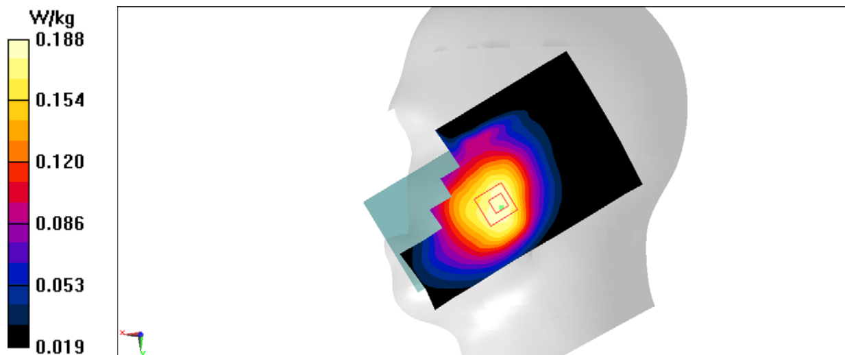
Fig.19 LTE Band5
