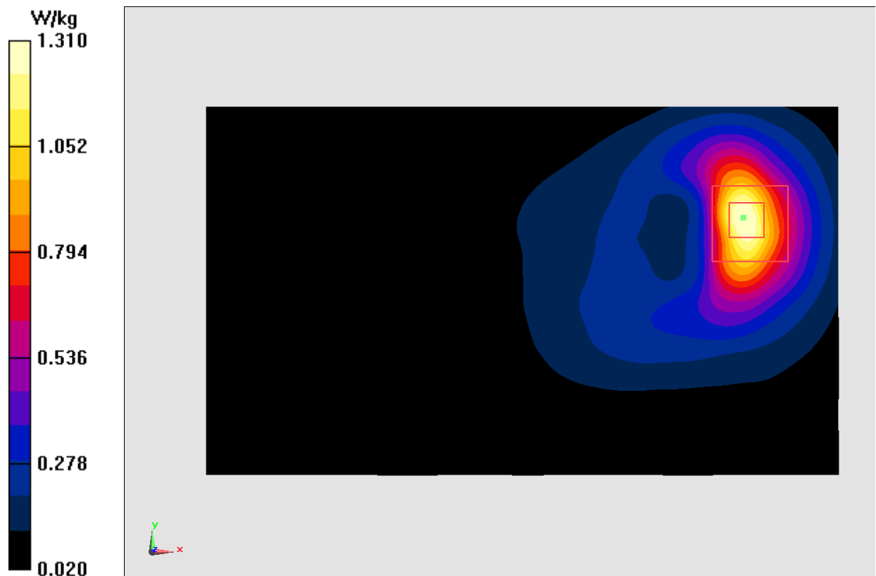
Fig.5 CDMA BC1
