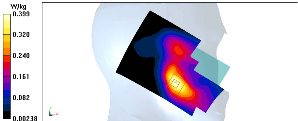
Fig.7 WCDMA1900
