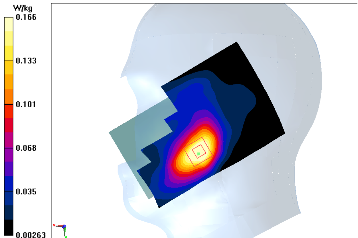
Fig.10 LTE Band2
