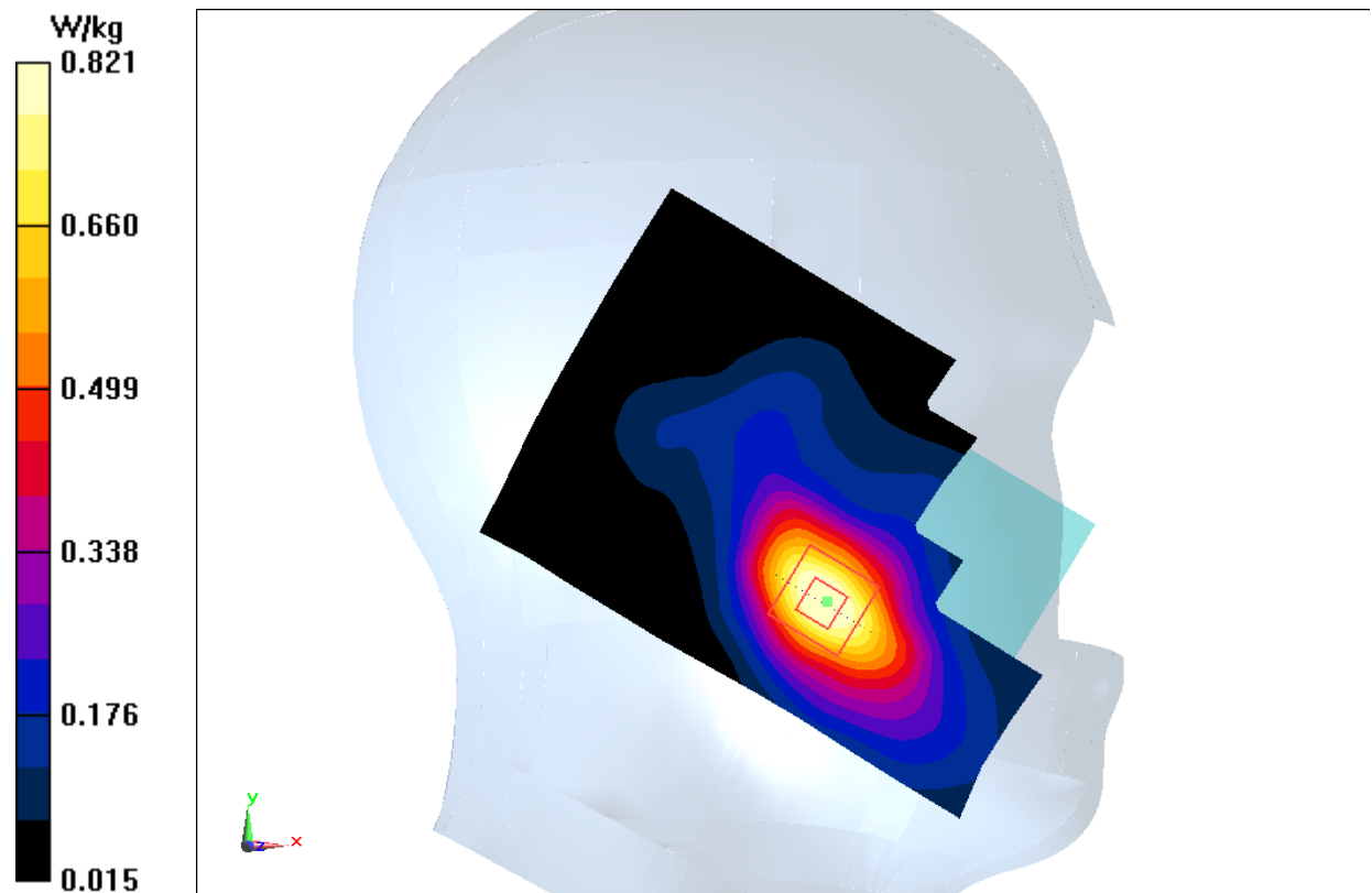
Fig.11 LTE Band2
