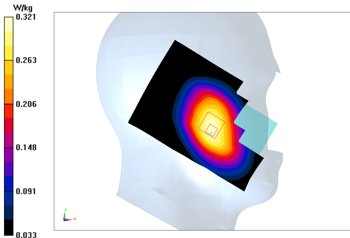
Fig.3 WCDMA 850
