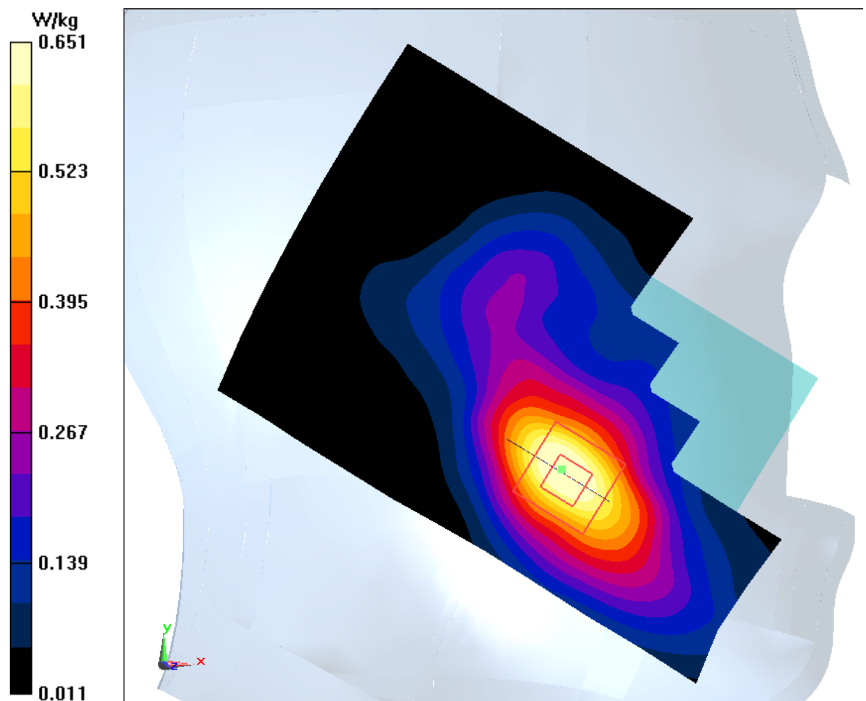
Fig.5 WCDMA1900
