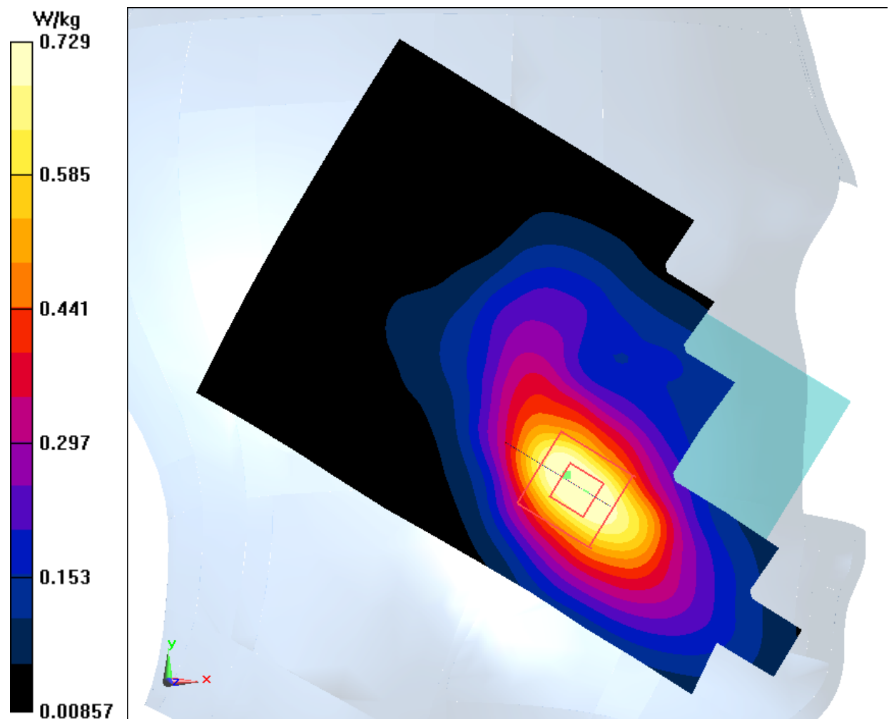
Fig.6 LTE Band2
