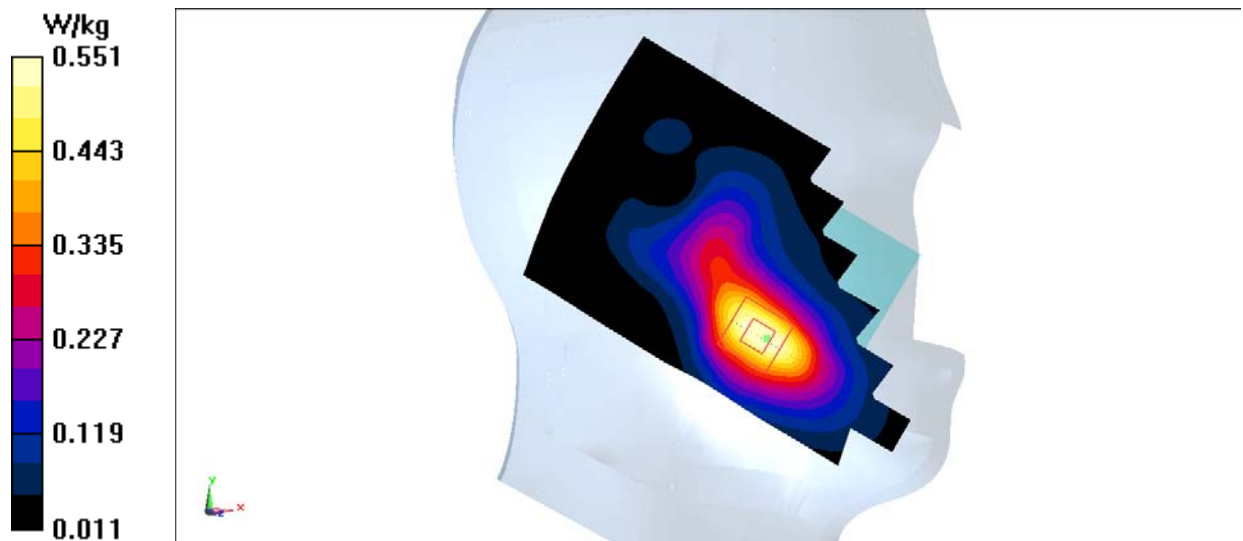
Fig.4 1700MHz
