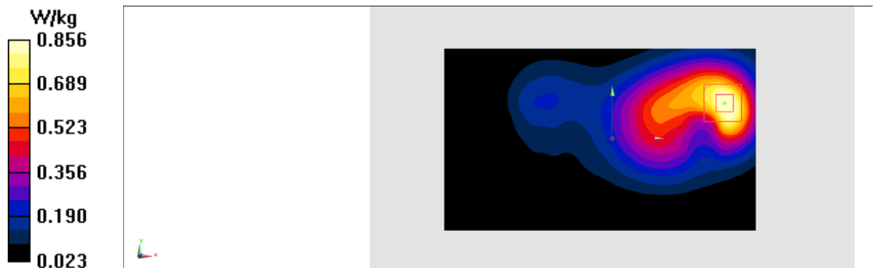
Fig.4 CDMA BC1
