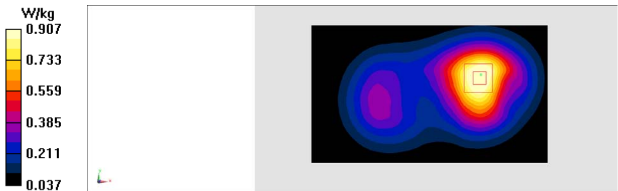
Fig.6 LTE Band4
