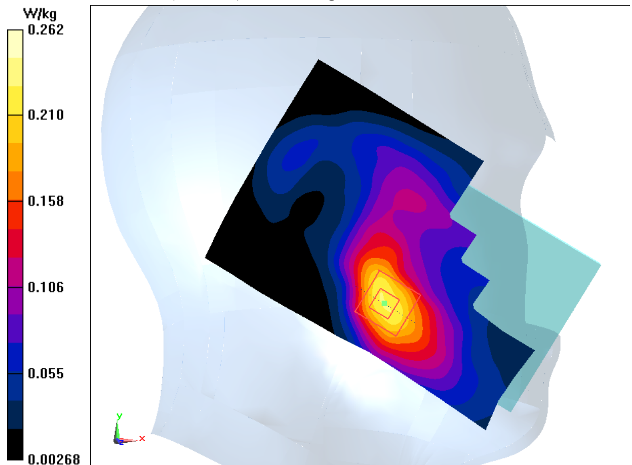
Fig.11 LTE Band4
