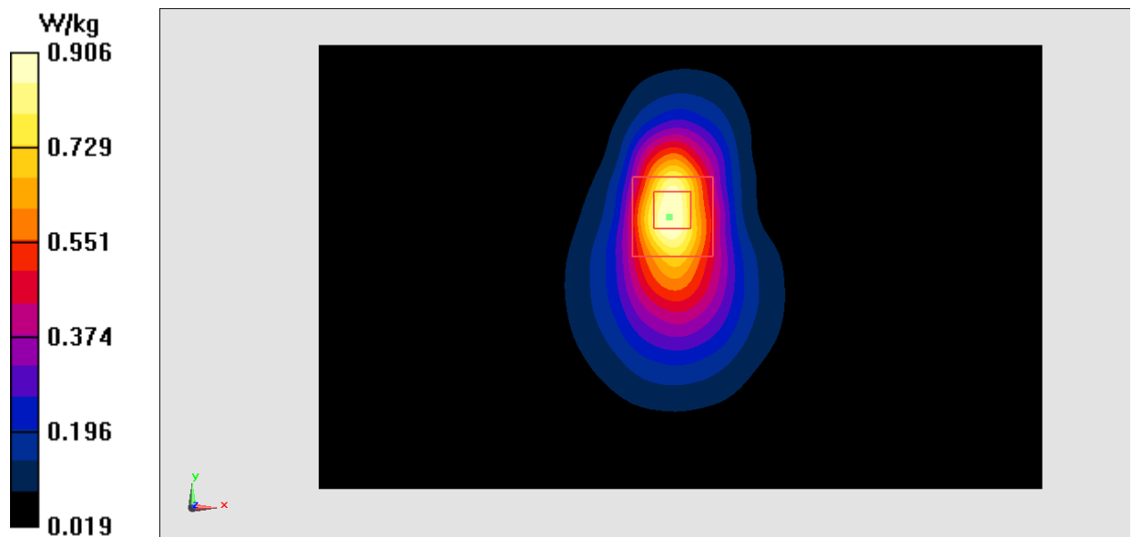
Fig.12 LTE Band4
