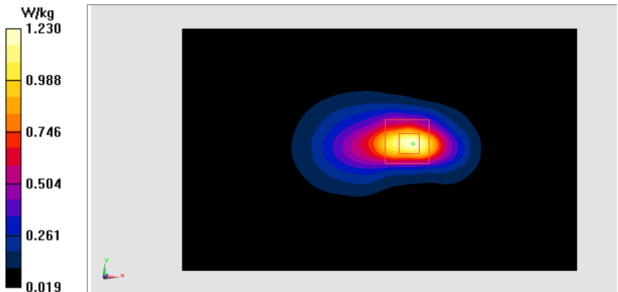
Fig.8 WCDMA1900
