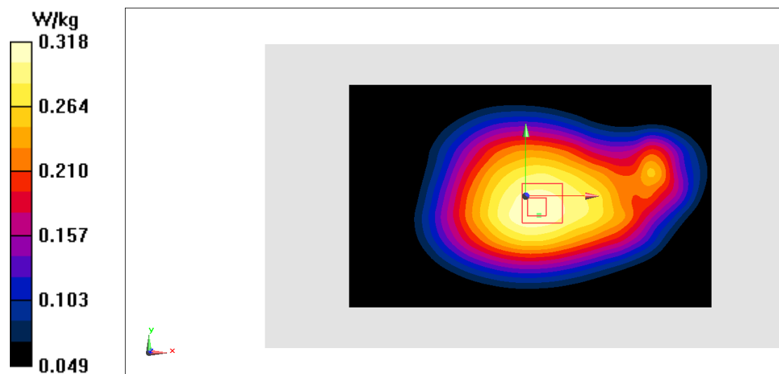
Fig.6 WCDMA 850
