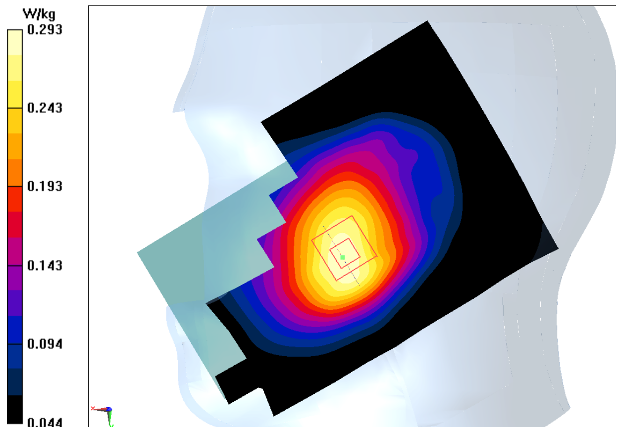
Fig.5 WCDMA 850
