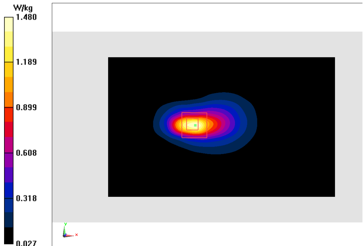
Fig.10 WCDMA1900
