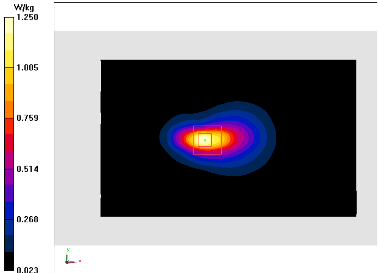
Fig.14 LTE Band4
