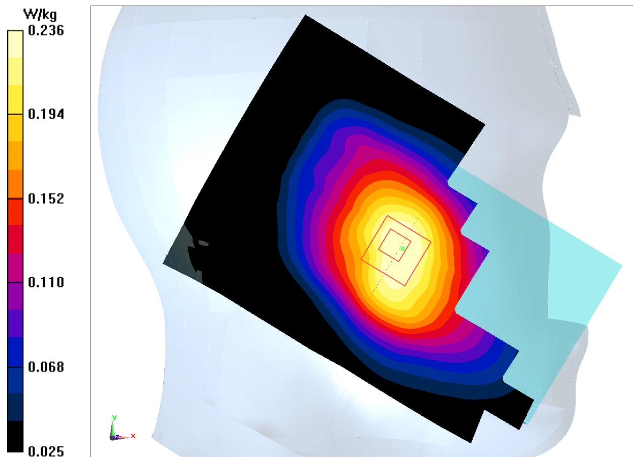
Fig.15 LTE Band5
