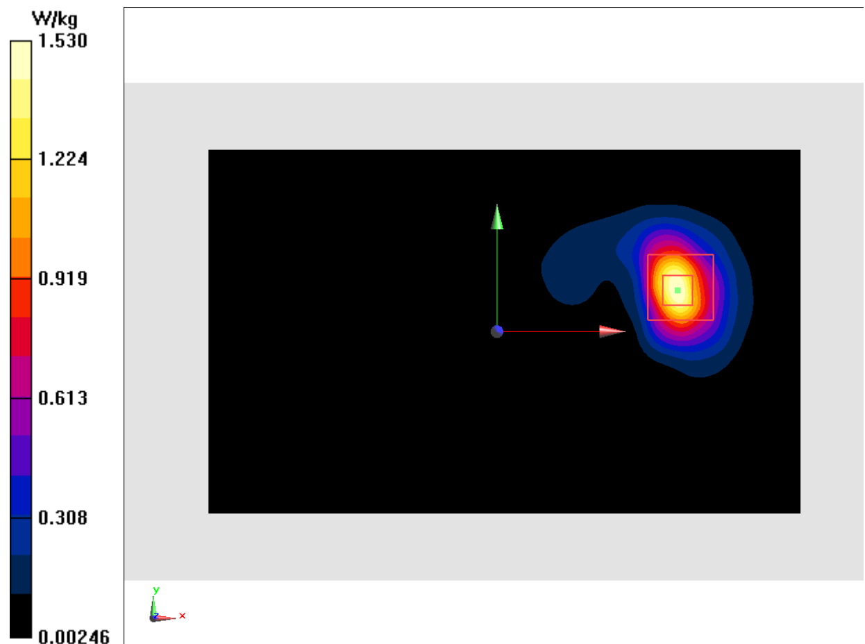
Fig.19 LTE Band7
