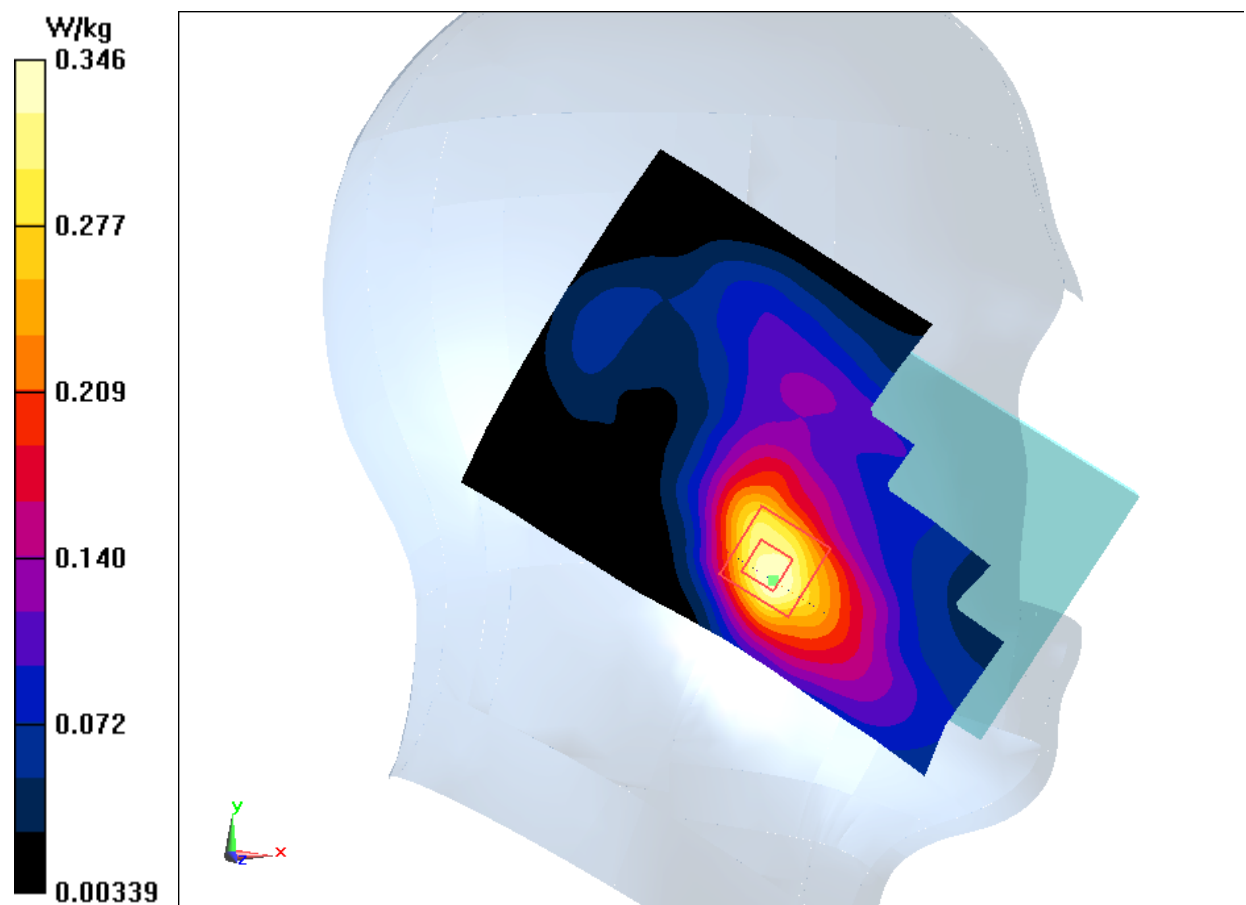
Fig.7 1700MHz
