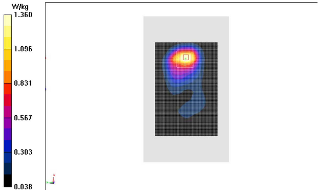
Fig.10 LTE Band2
