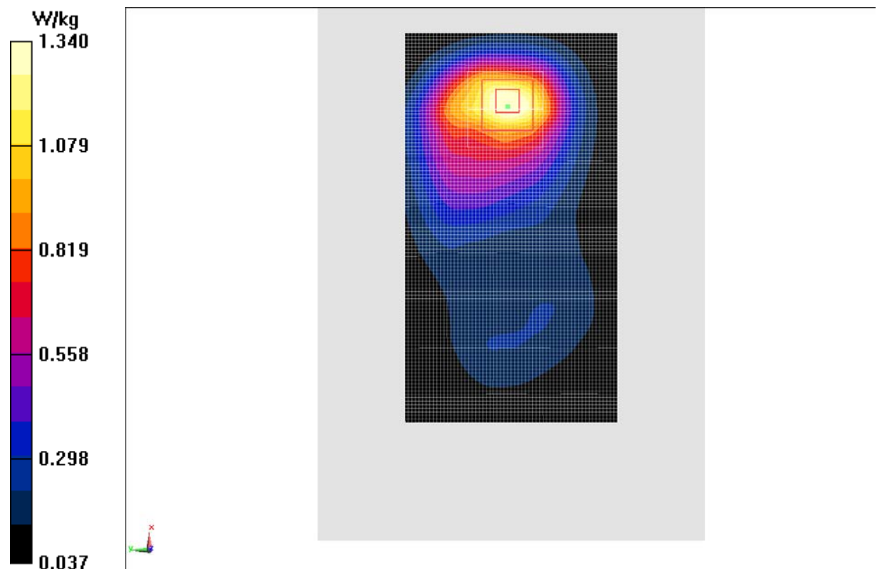
Fig.8 WCDMA1900
