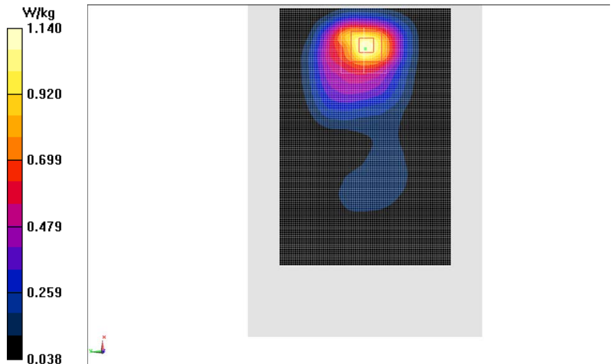
Fig.12 LTE Band4
