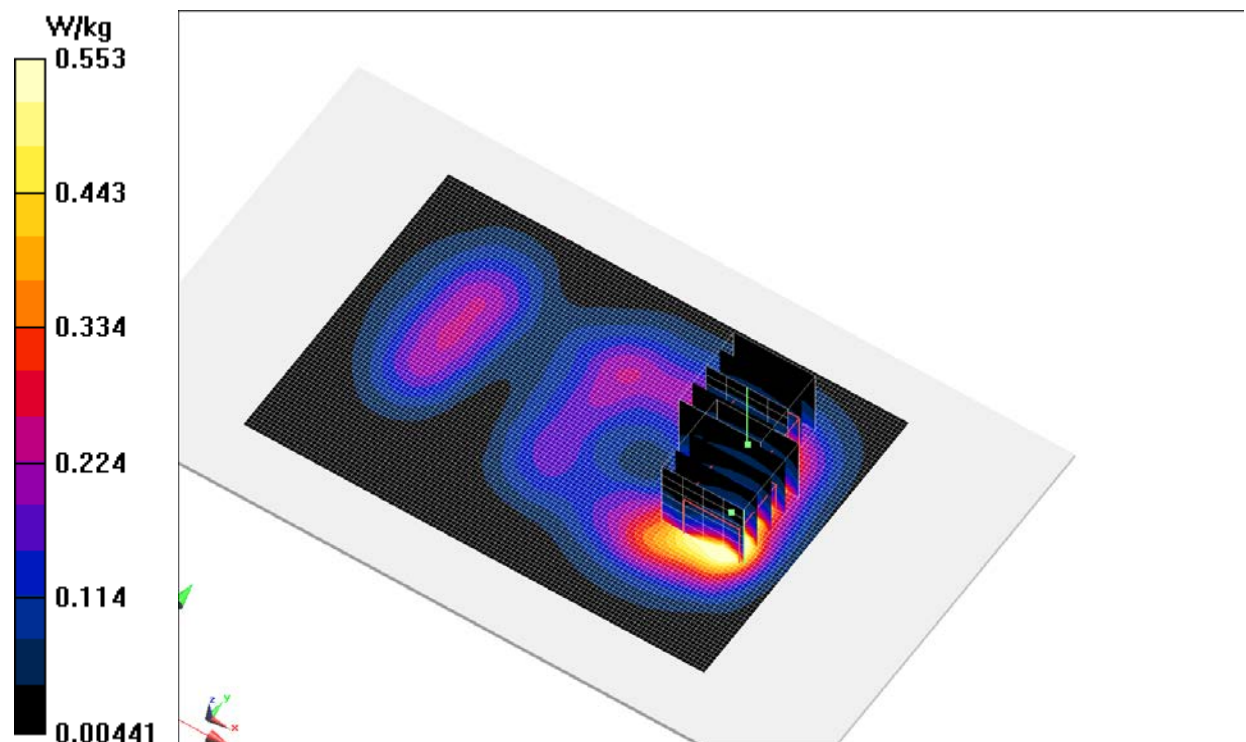
Fig.14 LTE Band7
