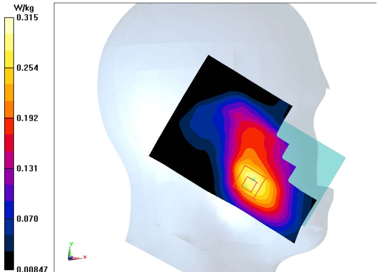
Fig.11 LTE Band4
