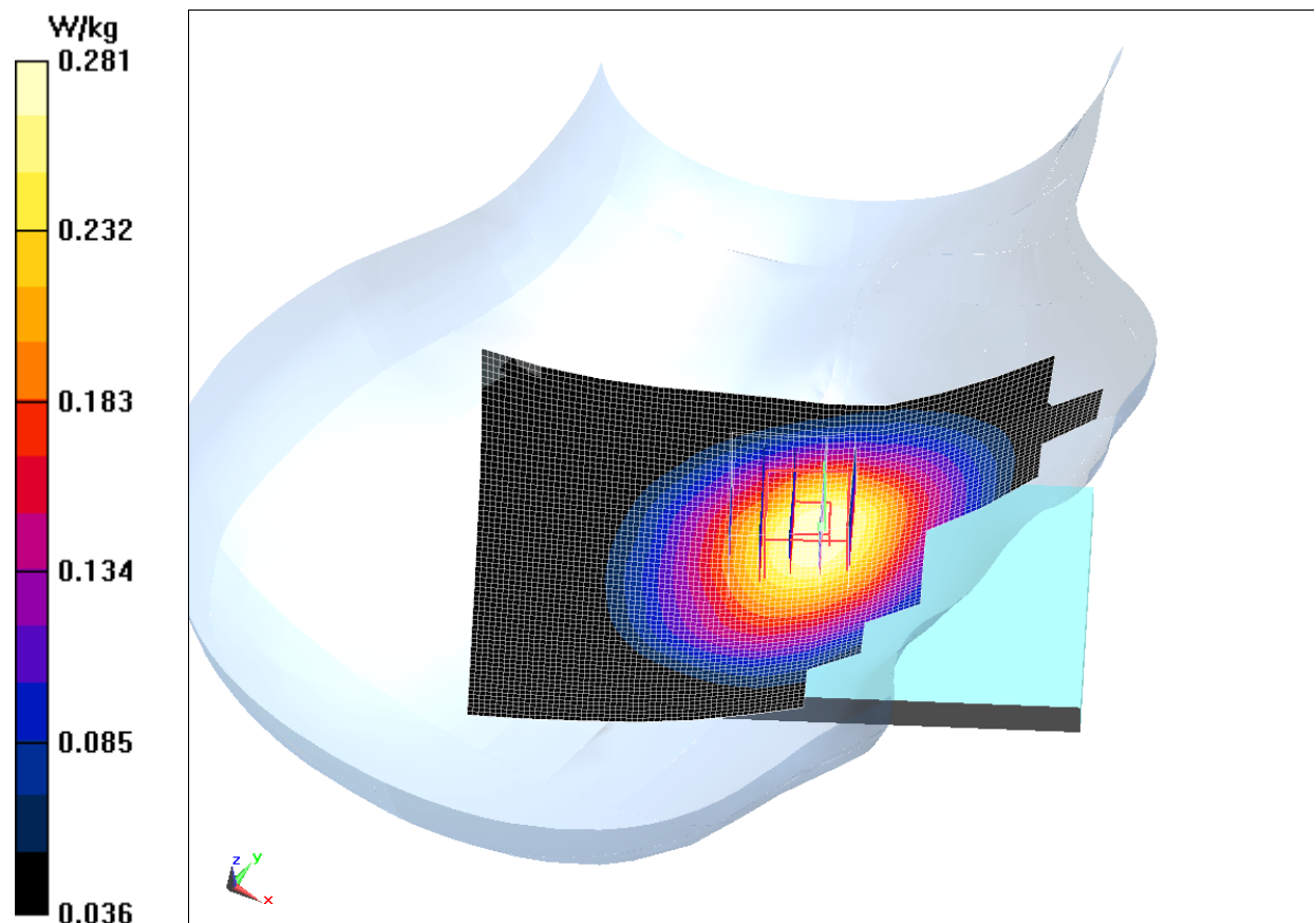
Fig.5 WCDMA 850
