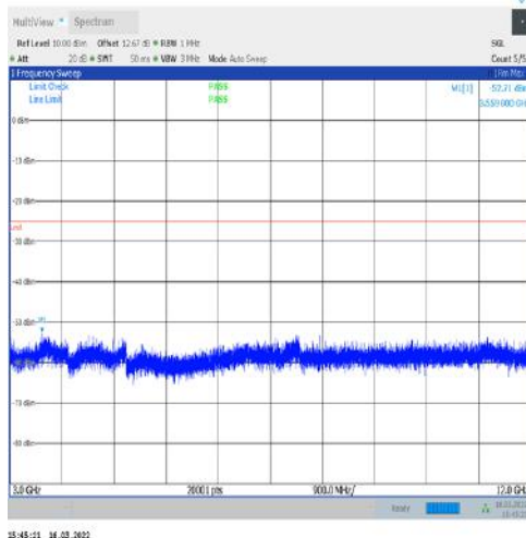
1-N41-3000-12000-Ant1--52.71--25-PASS
