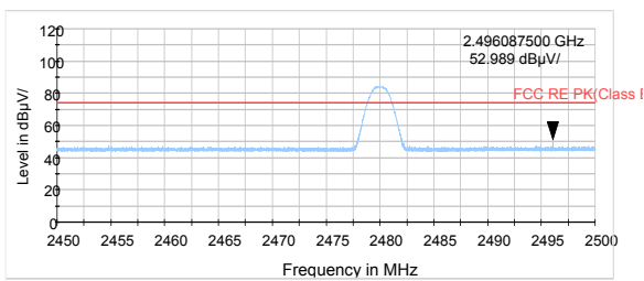
BLE Channel 39 Peak
