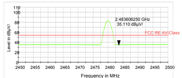
BLE Channel 39 Average
