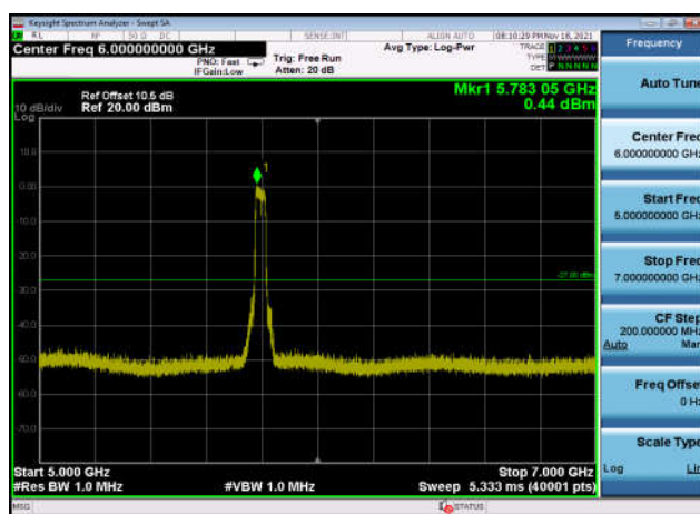
U-NII-3 ,Plot 3,5000MHz~7000MHz-802.1 1ac(40MHz),5795MHz,Ant1
