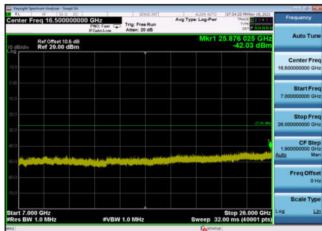
U-NII-3 ,Plot 4,7000MHz~26000MHz-802. 11ac(40MHz),5795MHz,Ant1
