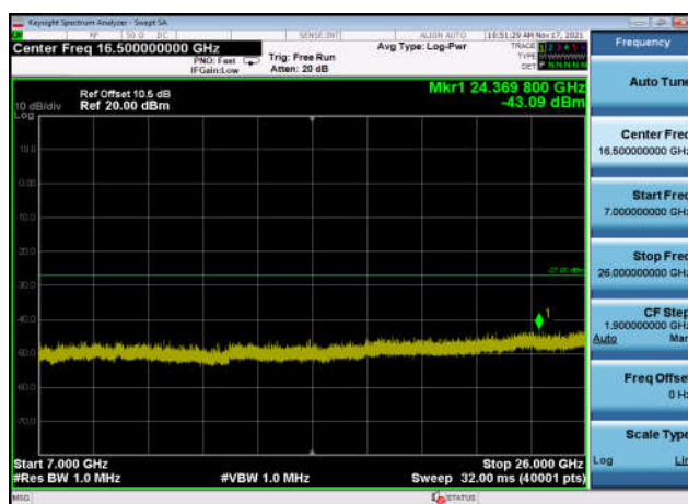
U-NII-3 ,Plot 4,7000MHz~26000MHz-802. 11ac(20MHz),5785MHz,Ant1
