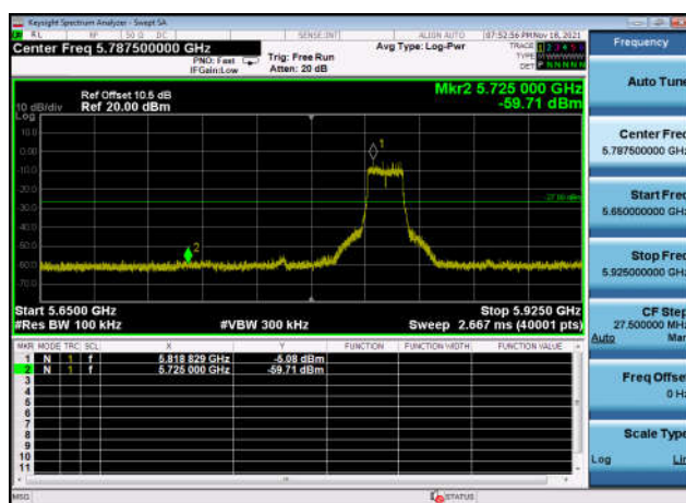
U-NII-3 ,Plot 1,Band Edge-802.11ac(40 MHz),5795MHz,Ant1
