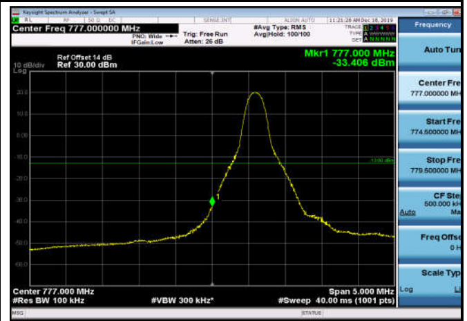
LowRange_FDD13_10MHz_782_OneRB_low_QPSK
