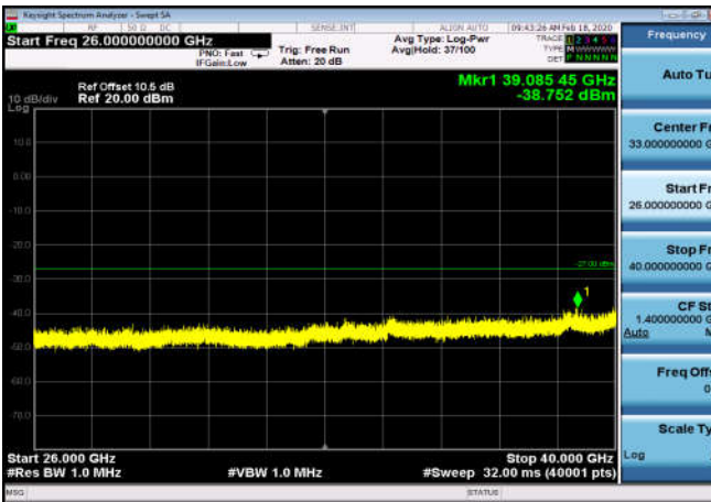
U-NII-1 ,Plot 5,26000MHz~40000MHz-802. 11a(20MHz),5180MHz,Ant1
