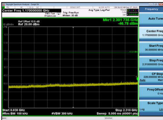
,Plot 3,30MHz~2310MHz-802.11b,2412MHz
