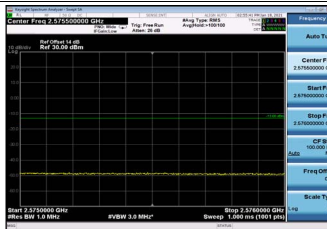
FDD07_20MHz_2560_QPSK_fullIRB_ExtraBan ds_Range_2575~2576
