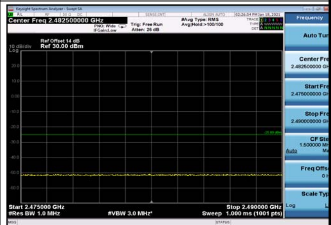
FDD07_5MHz_2567.5_QPSK_fullIRB_ExtraBa nds_Range_2475~2490
