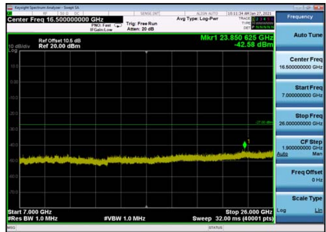
U-NII-2a ,Plot 4,7000MHz~26000MHz-802 .11ac(40MHz),5270MHz,Ant1
