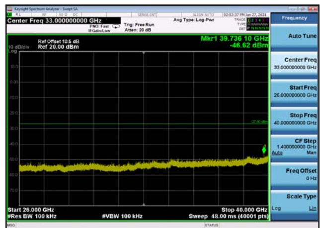
U-NII-2a ,Plot 2,26000MHz~40000MHz-80 2.11n(40MHz),5310MHz,Ant1
