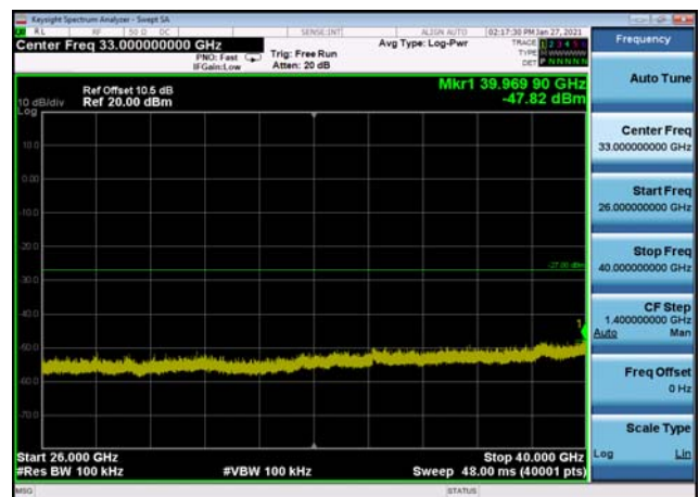
U-NII-2a ,Plot 2,26000MHz~40000MHz-80 2.11ac(20MHz),5300MHz,Ant1
