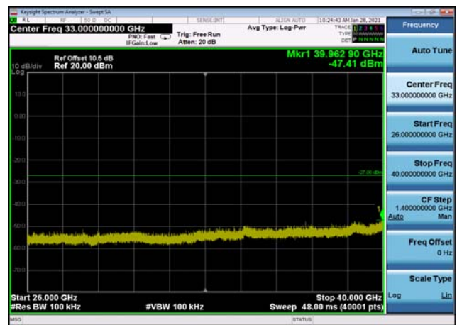
U-NII-3 ,Plot 2,26000MHz~40000MHz-802 .11n(20MHz),5825MHz,Ant1
