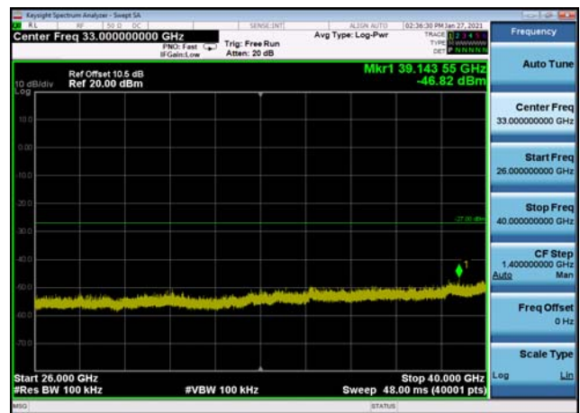
U-NII-2a ,Plot 2,26000MHz~40000MHz-80 2.11ac(20MHz),5300MHz,Ant1
