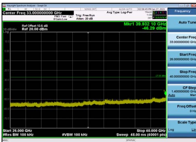
U-NII-2a ,Plot 2,26000MHz~40000MHz-80 2.11ac(40MHz),5310MHz,Ant1
