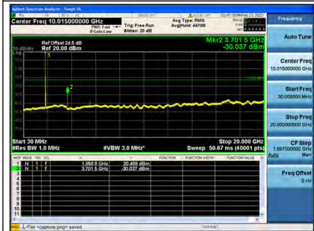
Band2 / 15MHz / Low CH / 64QAM
