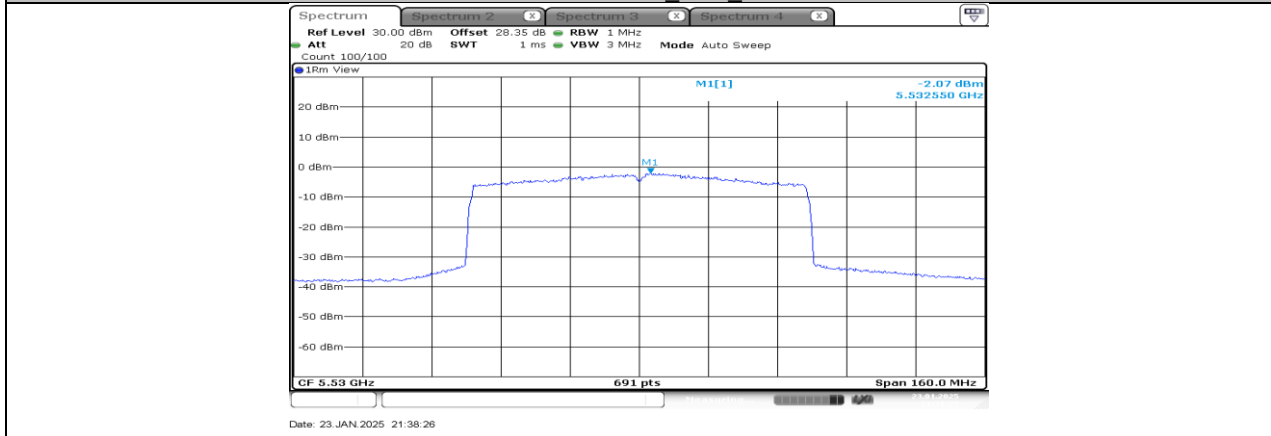
11AX80SISO SU_Ant3_5530
