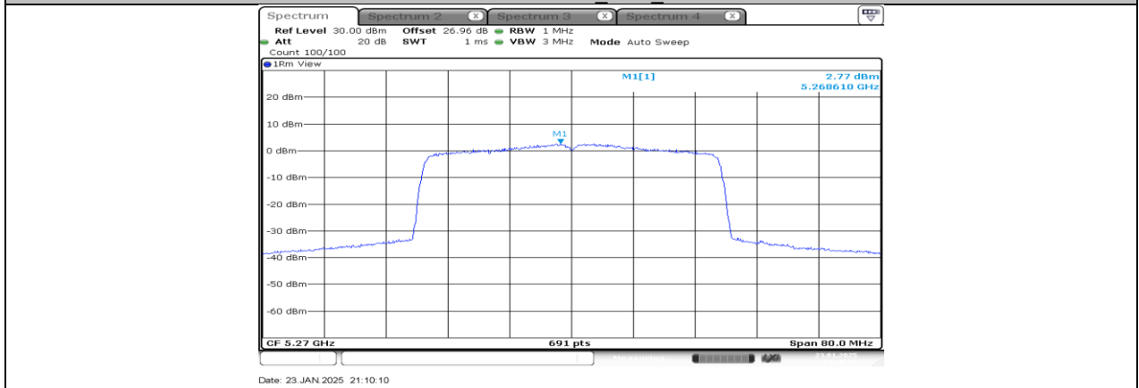
11AX40SISO SU_Ant3_5270
