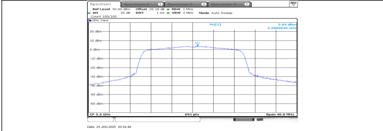
11AX20SISO SU_Ant3_5500
