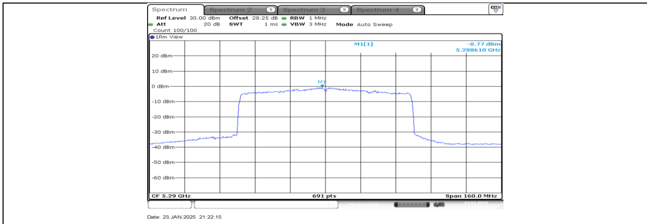
11AX80SISO SU_Ant3_5290
