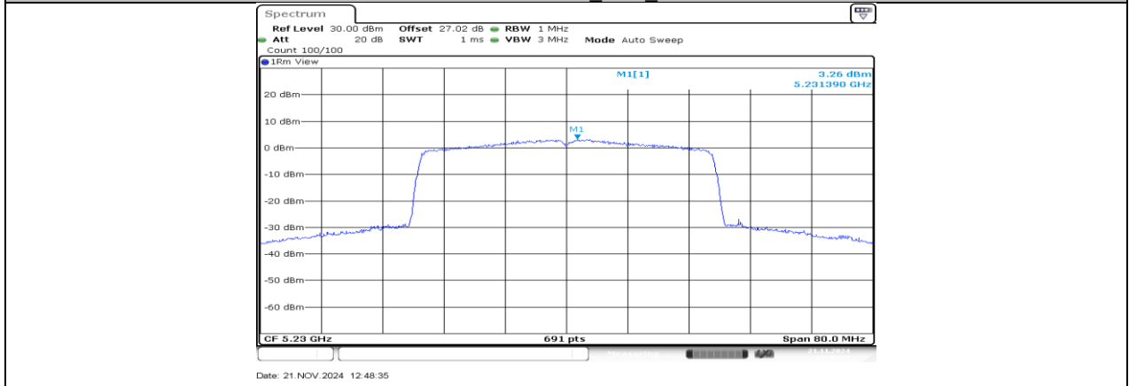
11AX40SISO SU_Ant3_5230
