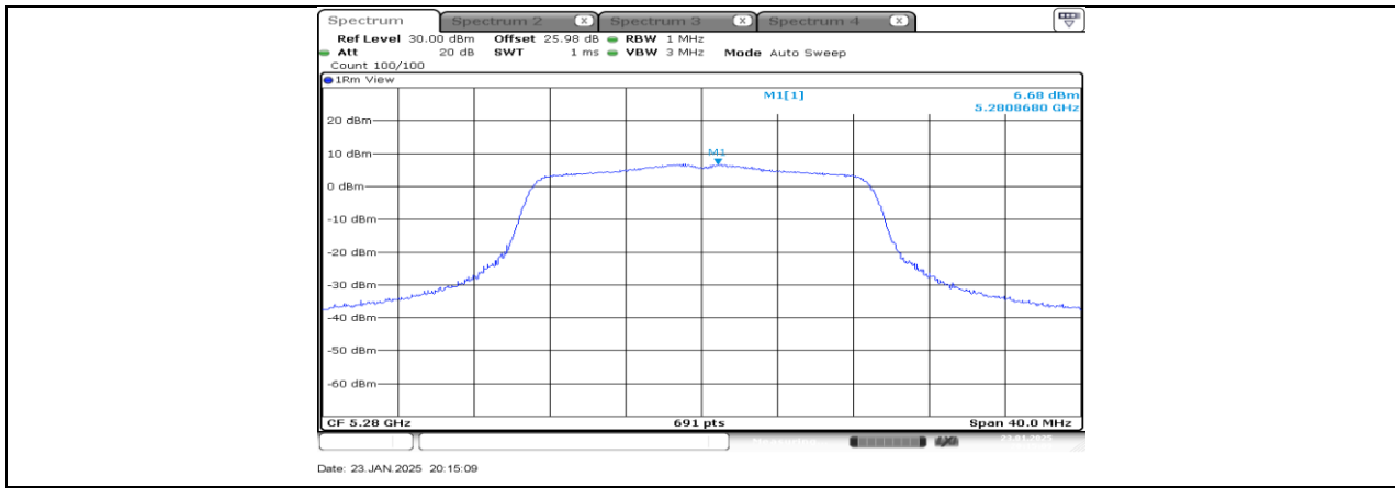
11N20SISO_Ant3_5280
