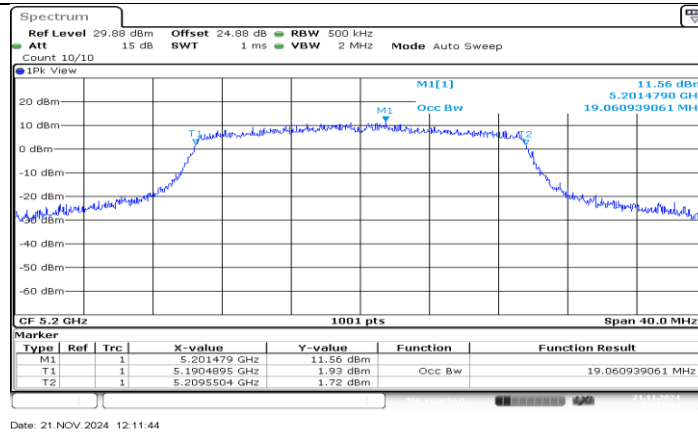
11AX20SISO SU_Ant3_5200
