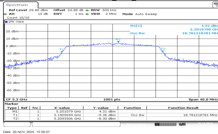
11N20SISO_Ant3_5200
