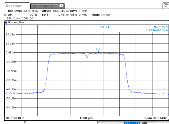
n40_5230MHz_Chain 1
