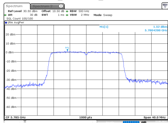
ac20_5785MHz_Chain 1
