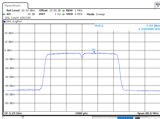
n40_5230MHz_Chain 0
