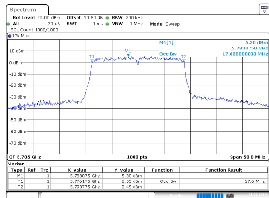
ac20_5785MHz_Chain 0
