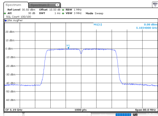
n40_5190MHz_Chain 1
