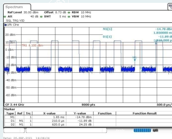
BLE_2M_2440
