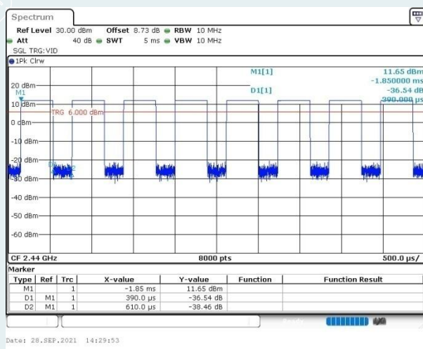
BLE_1M_2440
