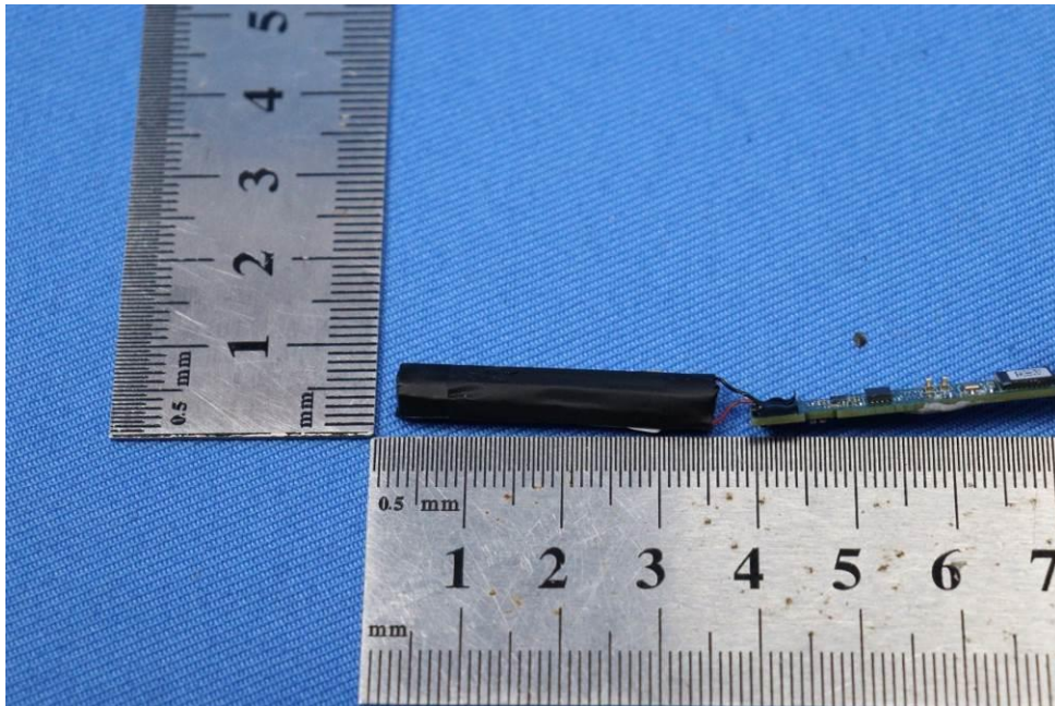
BLE Antenna Location
