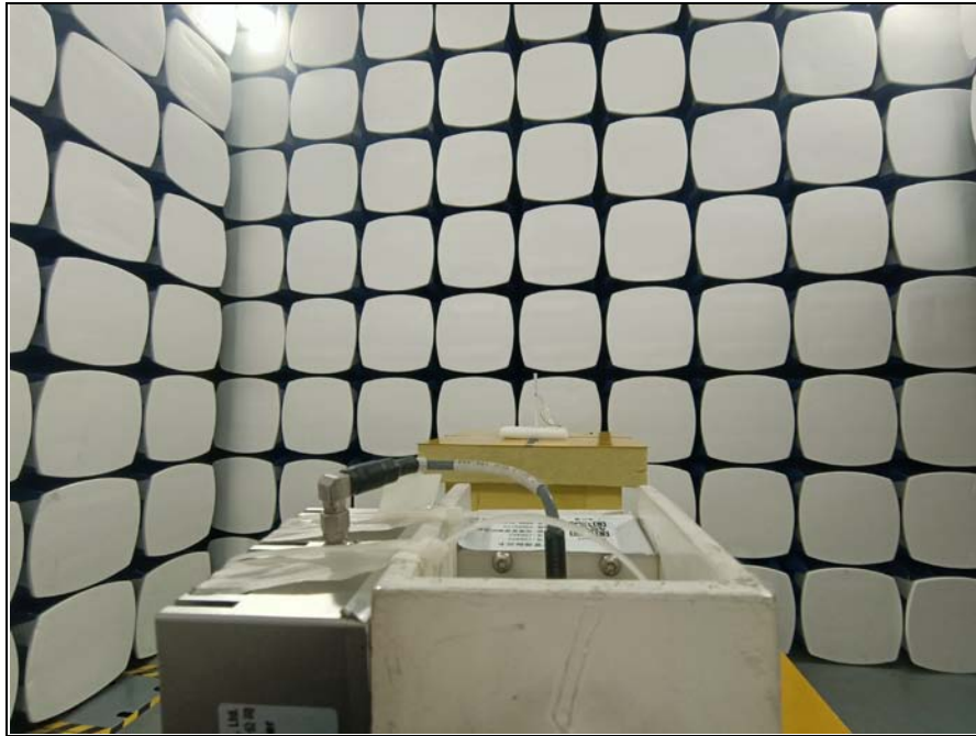
18GHz-26.5GHz
