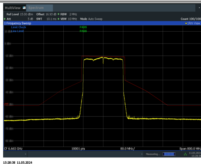
11BE160MIMO_Ant1_6665
