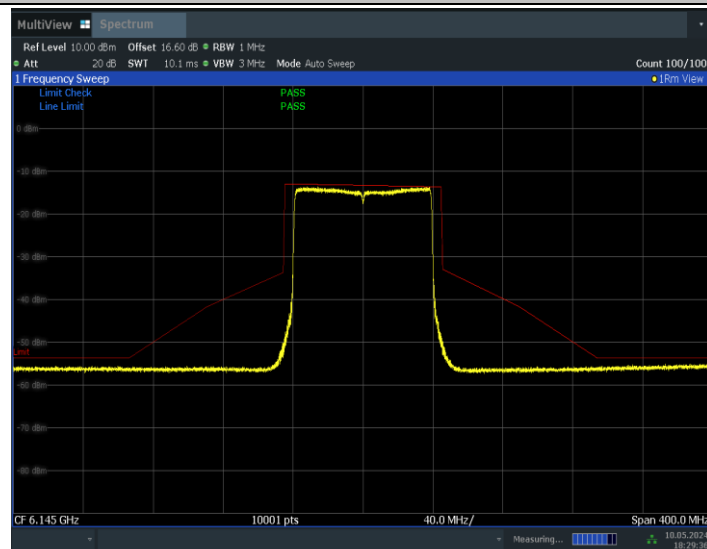
11BE80MIMO_Ant1_6145
