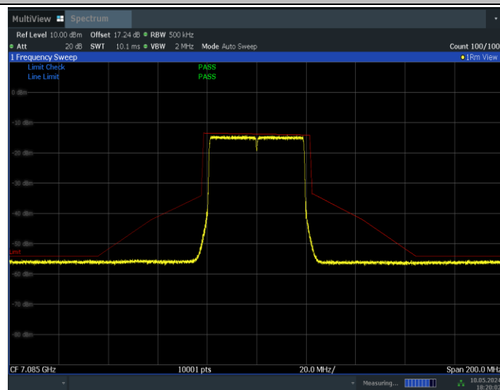
11BE40MIMO_Ant0_7085
