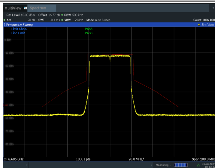
11BE40MIMO_Ant0_6685
