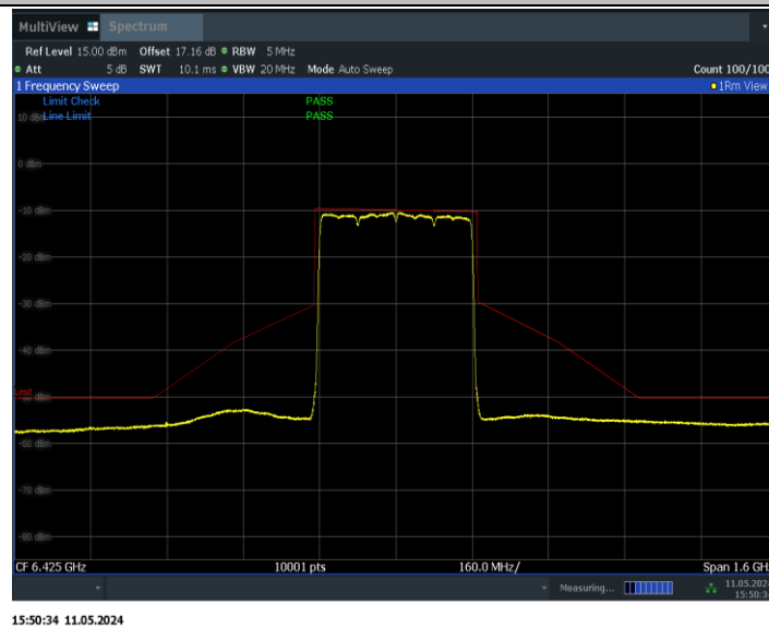
11BE320MIMO_Ant1_6425
