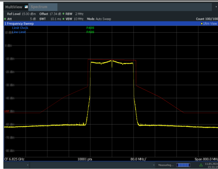
11BE160MIMO_Ant0_6825
