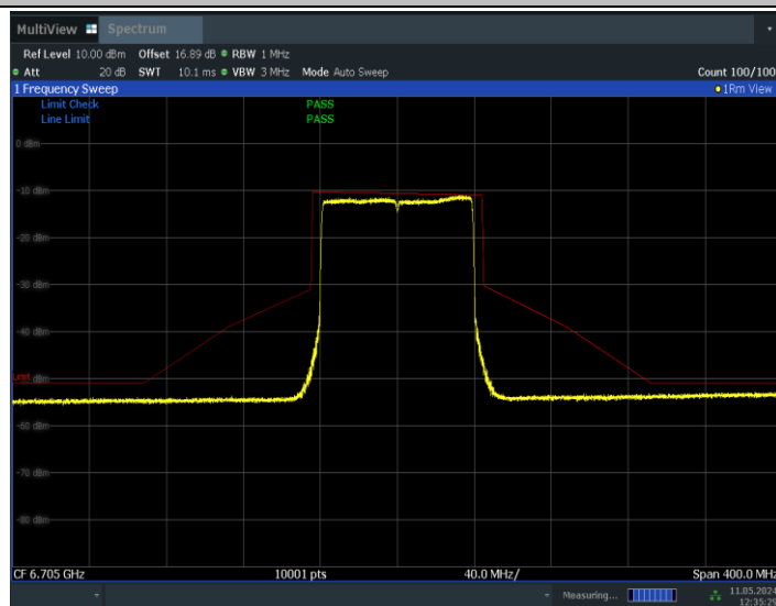
11BE80MIMO_Ant1_6705
