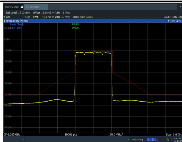
11BE320MIMO_Ant0_6265
