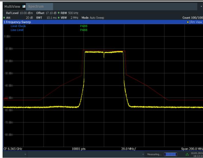
11BE40MIMO_Ant1_6565
