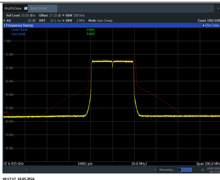
11BE40MIMO_Ant1_6925
