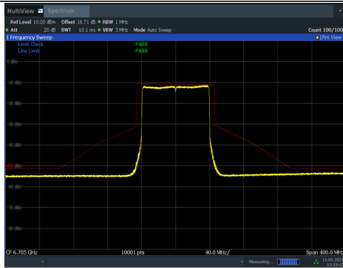
11BE80MIMO_Ant0_6705
