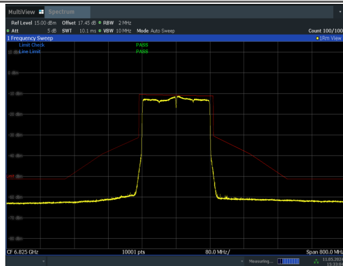
11BE160MIMO_Ant1_6825
