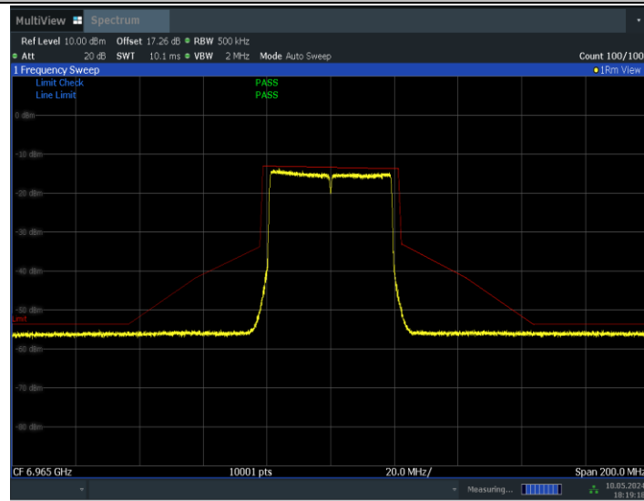
11BE40MIMO_Ant1_6965
