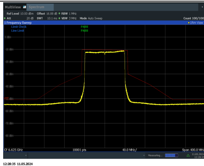
11BE80MIMO_Ant1_6625
