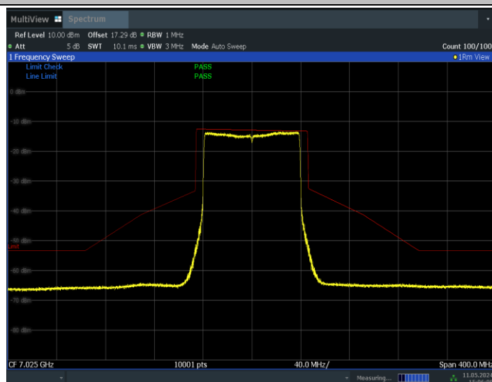
11BE80MIMO_Ant1_7025
