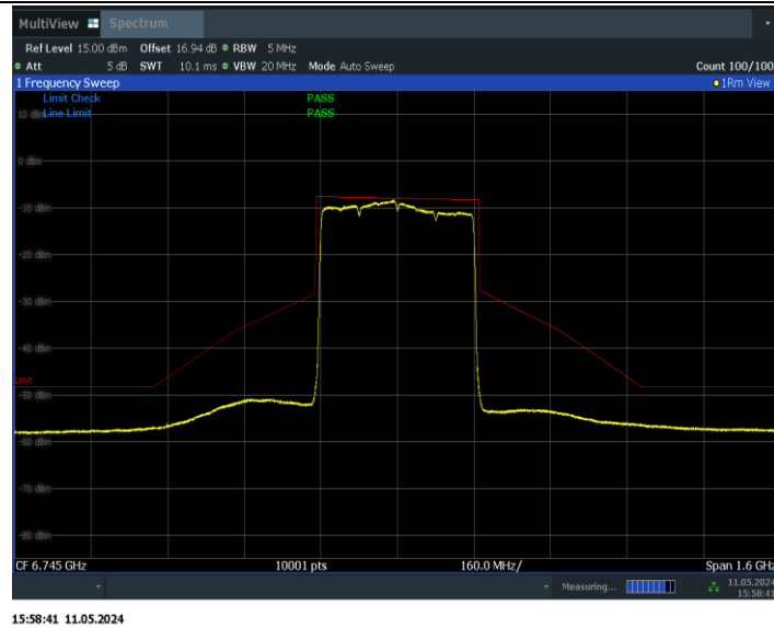
11BE320MIMO_Ant1_6745
