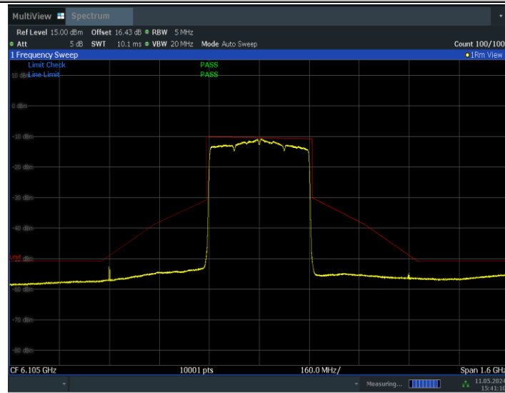
11BE320MIMO_Ant1_6105
