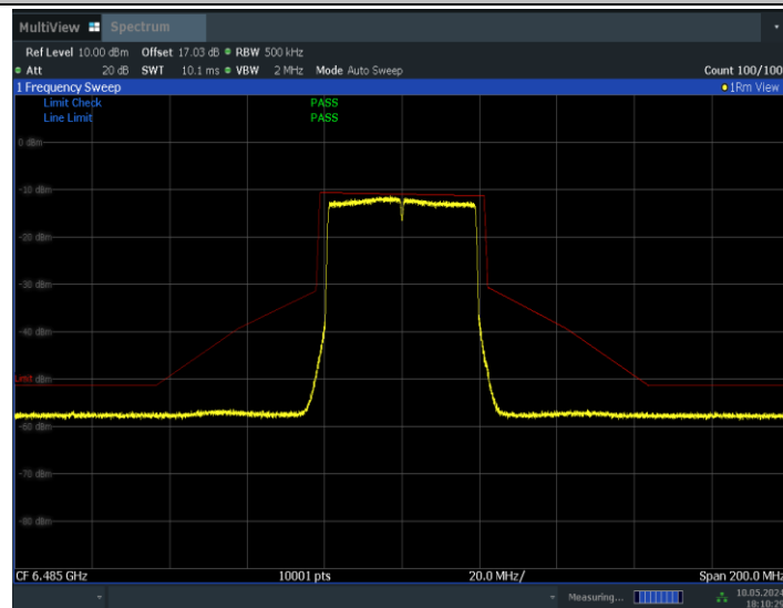
11BE40MIMO_Ant1_6485
