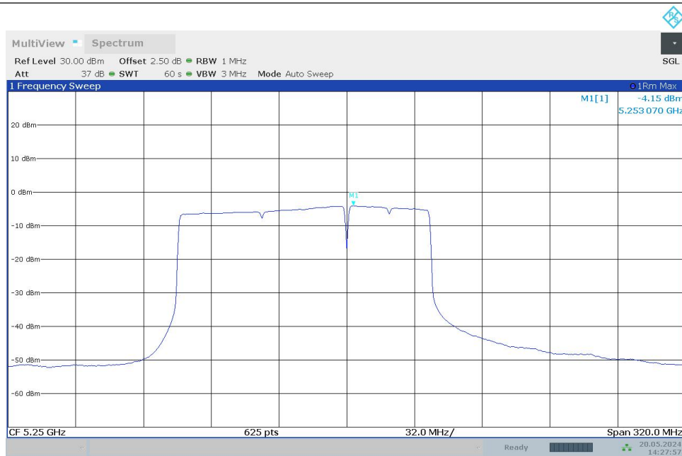
11BE160MIMO_Ant0_5250_996+484+242_OFDMA_1
