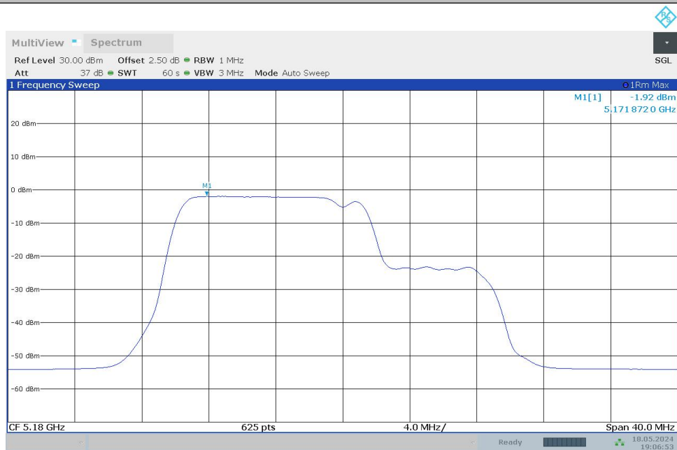
11BE20MIMO_Ant1_5180_106+26_OFDMA_1
