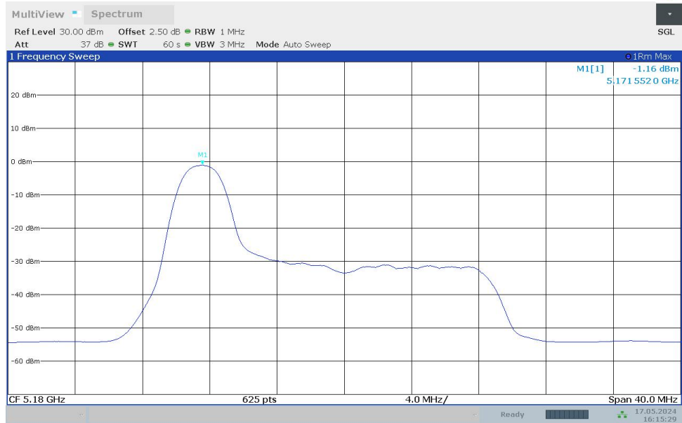
11AX20MIMO_Ant0_5180_52Tone_RU37
