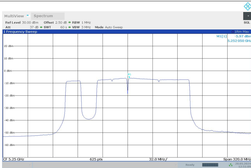
11BE160MIMO_Ant0_5250_996+484+242_OFDMA_3
