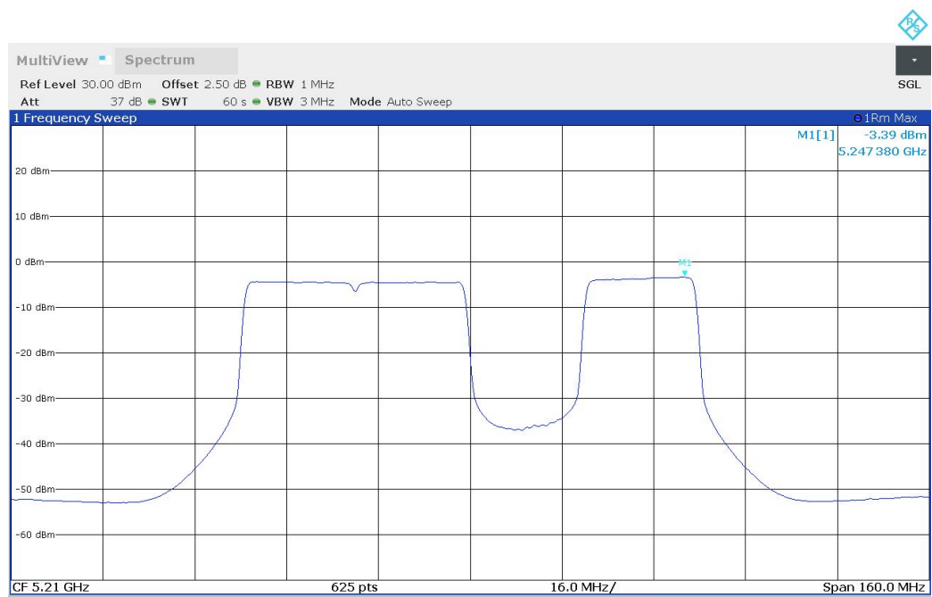
11BE80MIMO_Ant1_5210_484+242_OFDMA_4
