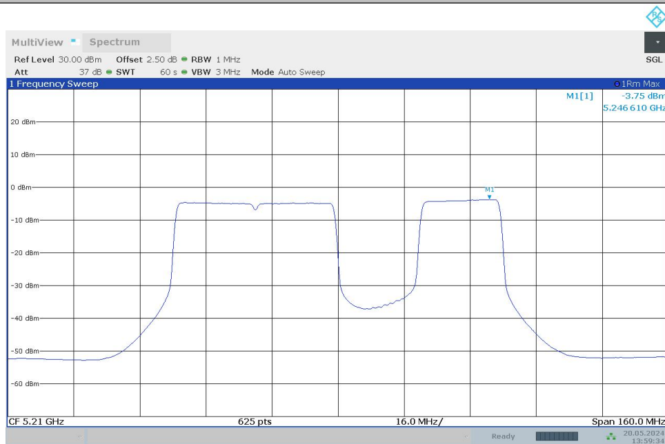
11BE80MIMO_Ant0_5210_484+242_OFDMA_3
