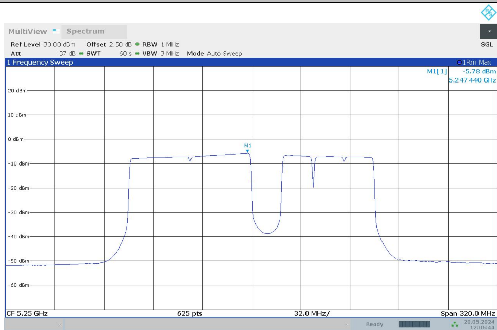
11BE160MIMO_Ant1_5250_996+484+242_OFDMA_5
