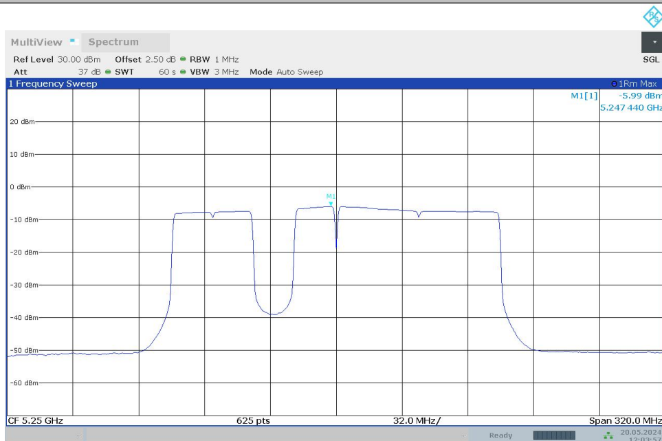
11BE160MIMO_Ant1_5250_996+484+242_OFDMA_3
