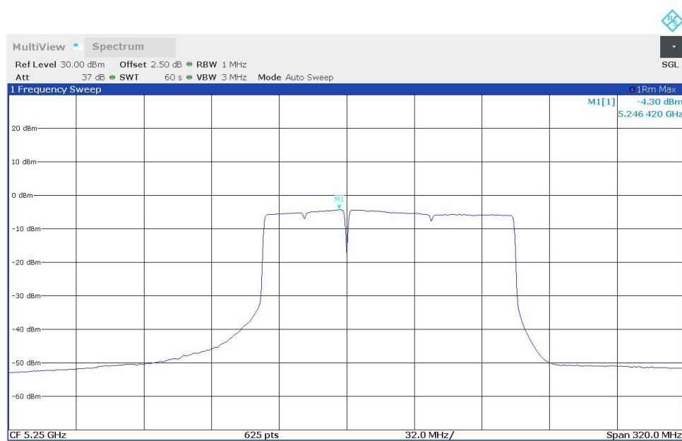
11BE160MIMO_Ant1_5250_996+484_OFDMA_2
