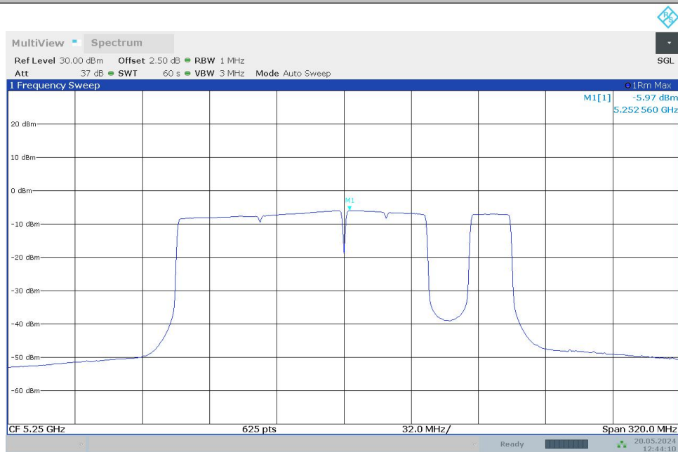
11BE160MIMO_Ant0_5250_996+484+242_OFDMA_7
