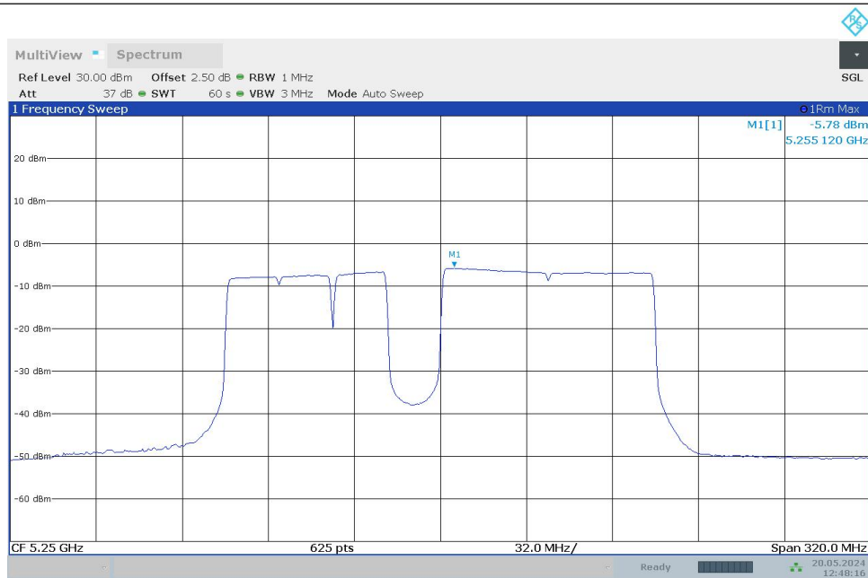
11BE160MIMO_Ant0_5250_996+484+242_OFDMA_5
