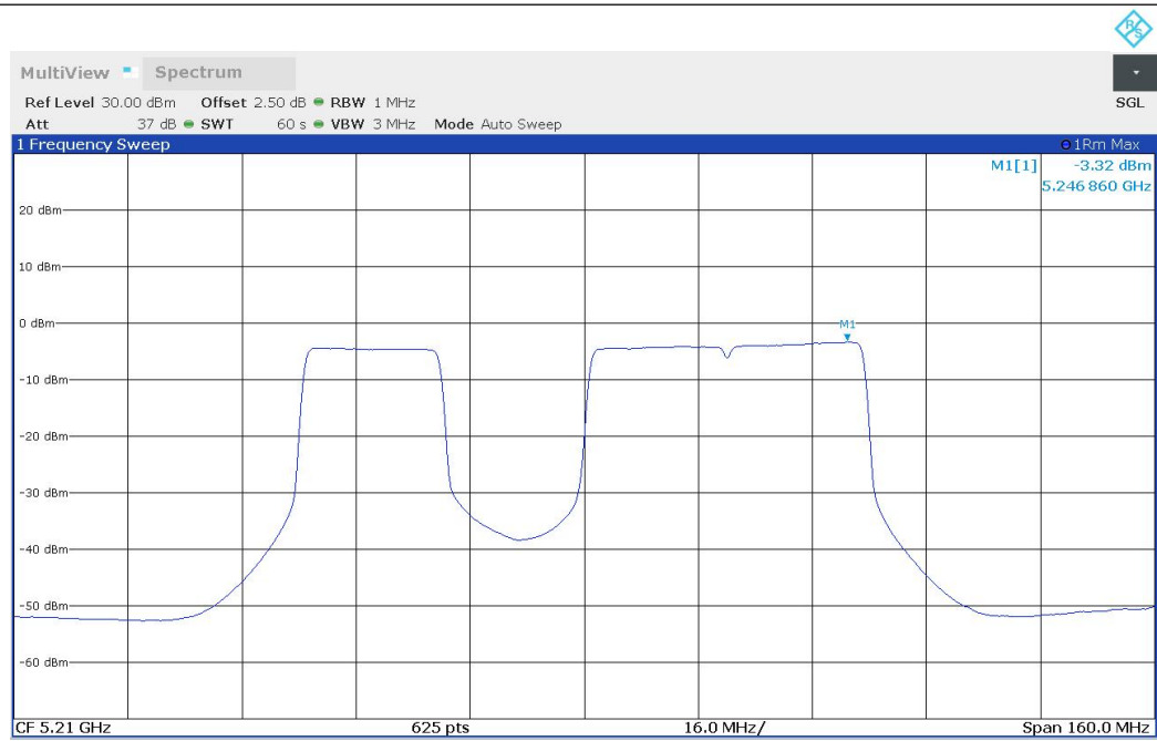
11BE80MIMO_Ant1_5210_484+242_OFDMA_3
