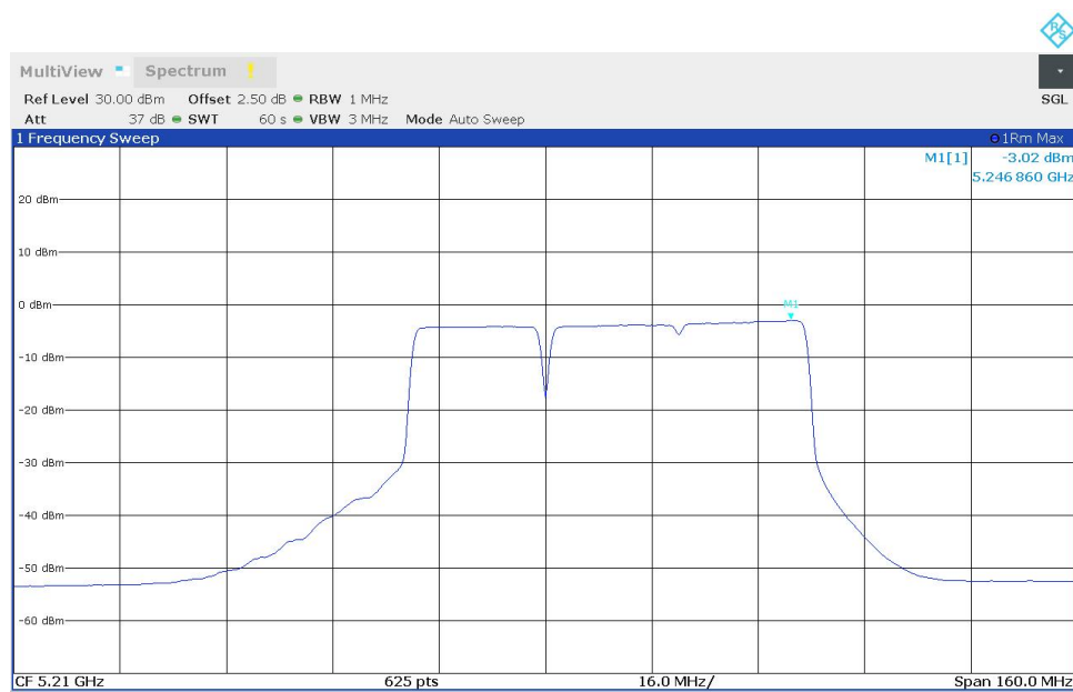
11BE80MIMO_Ant1_5210_484+242_OFDMA_2
