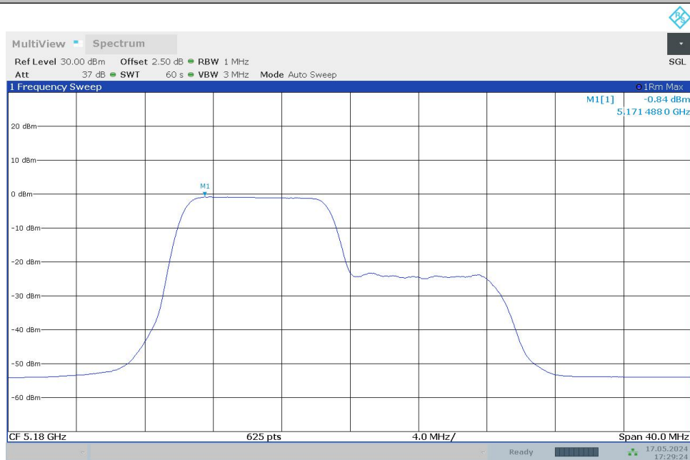
11AX20MIMO_Ant0_5180_106Tone_RU53
