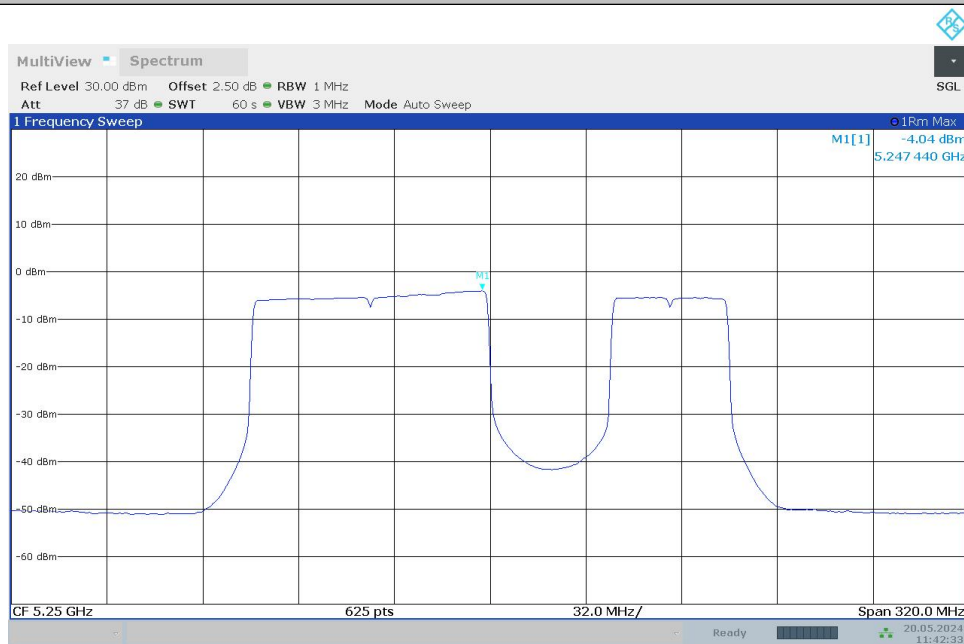
11BE160MIMO_Ant1_5250_996+484_OFDMA_3
