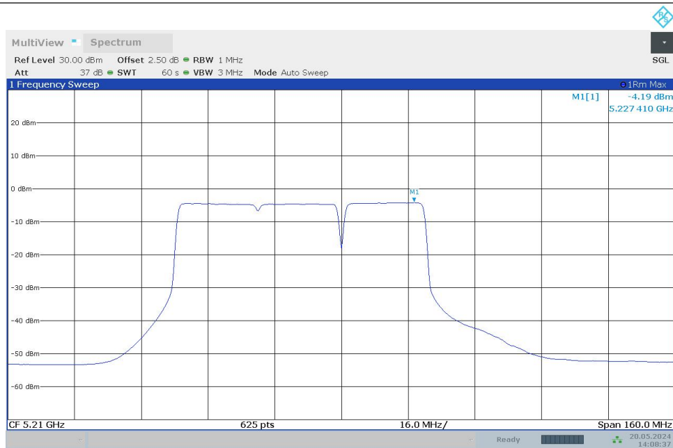
11BE80MIMO_Ant1_5210_484+242_OFDMA_1
