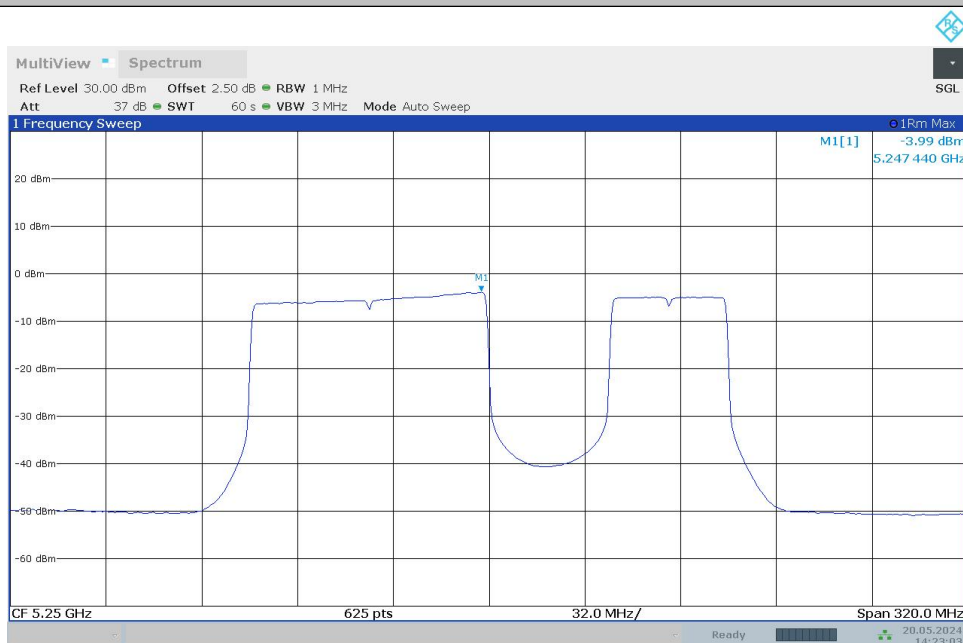
11BE160MIMO_Ant0_5250_996+484_OFDMA_3
