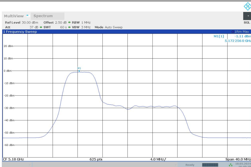
11AX20MIMO_Ant1_5180_52Tone_RU37
