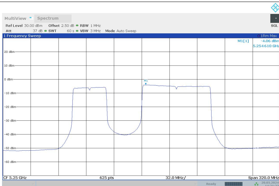
11BE160MIMO_Ant0_5250_996+484_OFDMA_3
