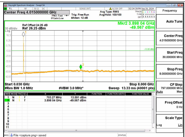
12B / 5+10MHz / QPSK / Mid CH / 25@0-50@0
