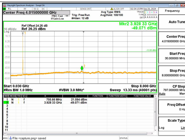
12B / 5+10MHz / QPSK / Mid CH / 1@24-1@0
