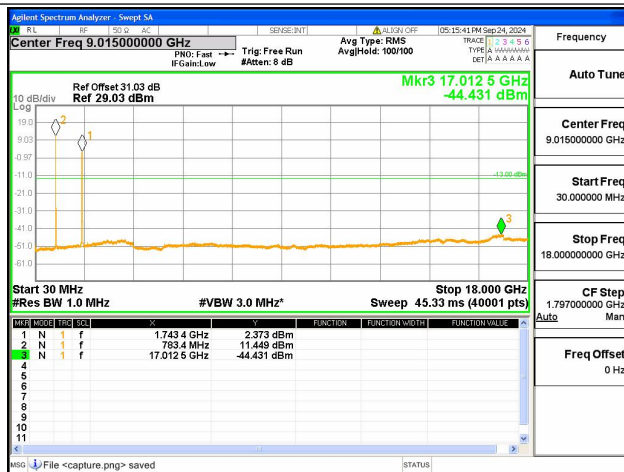
13A-66A / 10+20MHz / QPSK / Low+Mid CH / 50@0-100@0
