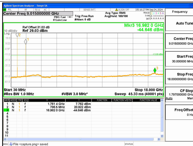
13A-66A / 10+20MHz / QPSK / Low+High CH / 1@49-1@0
