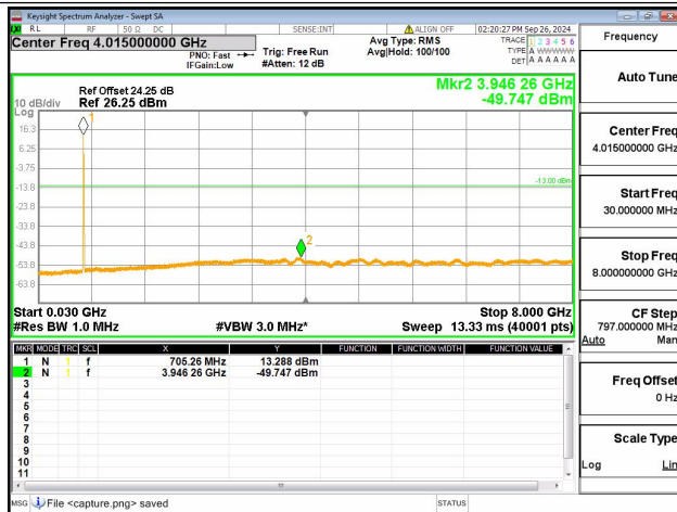
12B / 5+5MHz / QPSK / Mid CH / 25@0-25@0
