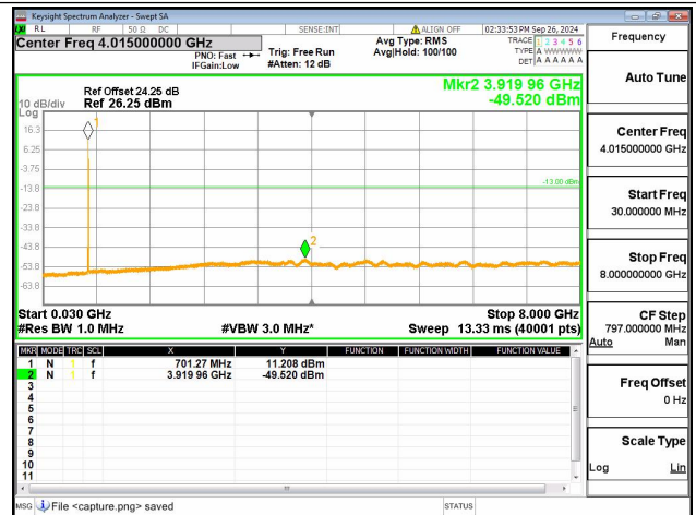
12B / 5+10MHz / QPSK / Mid CH / 1@0-1@49
