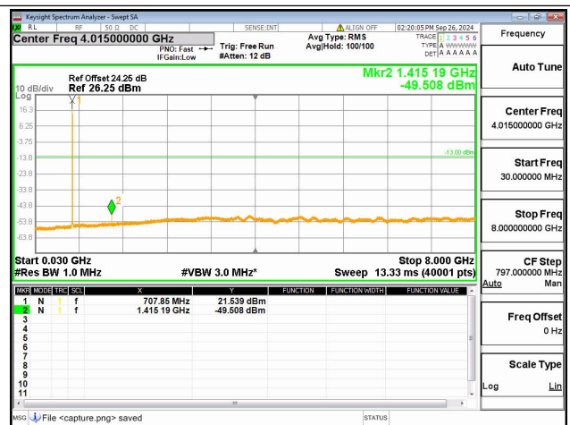
12B / 5+5MHz / QPSK / Mid CH / 1@24-1@0
