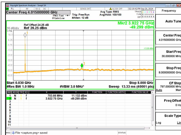
12B / 5+5MHz / QPSK / Mid CH / 1@0-1@24
