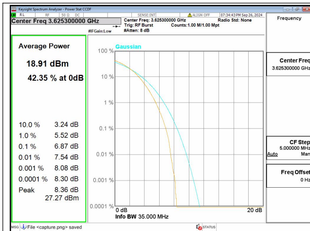
48C / 15+20MHz / Mid CH / 64QAM
