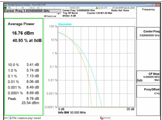
48C / 10+20MHz / Mid CH / 256QAM
