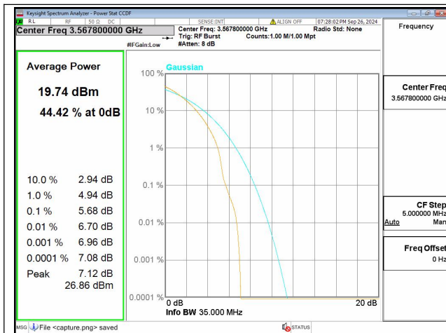
48C / 15+20MHz / Low CH / QPSK
