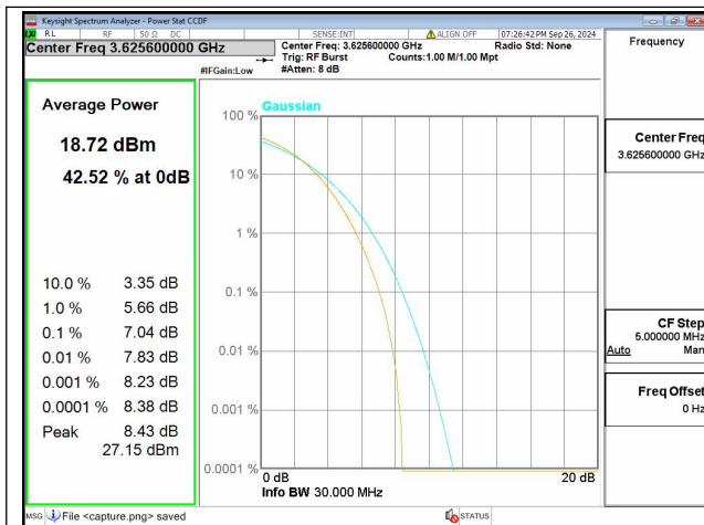
48C / 10+20MHz / Mid CH / 64QAM
