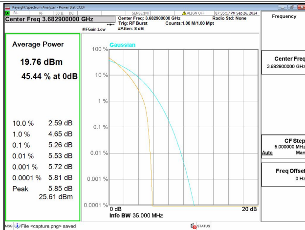
48C / 15+20MHz / High CH / QPSK
