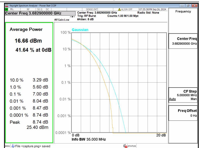
48C / 15+20MHz / High CH / 256QAM
