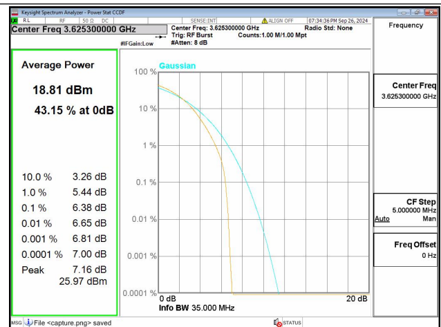
48C / 15+20MHz / Mid CH / 16QAM
