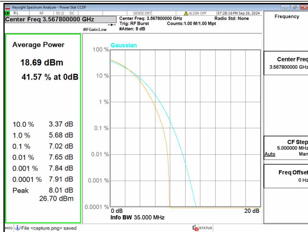
48C / 15+20MHz / Low CH / 64QAM
