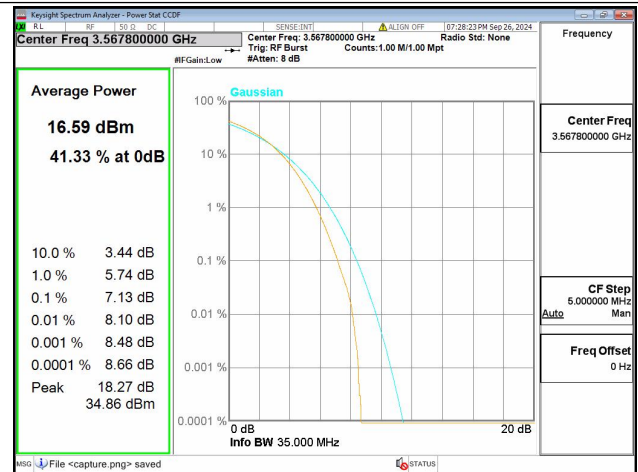
48C / 15+20MHz / Low CH / 256QAM
