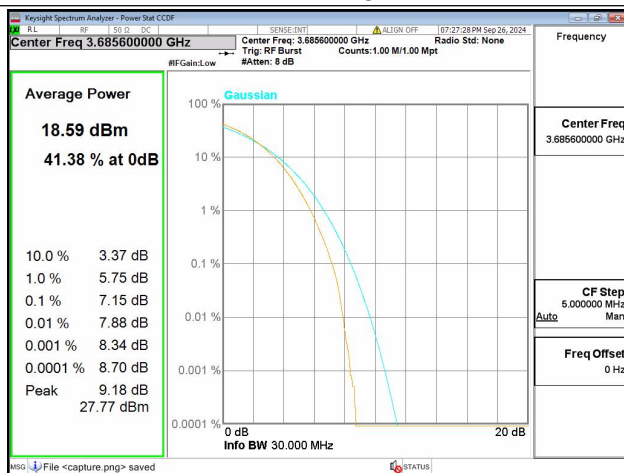
48C / 10+20MHz / High CH / 64QAM
