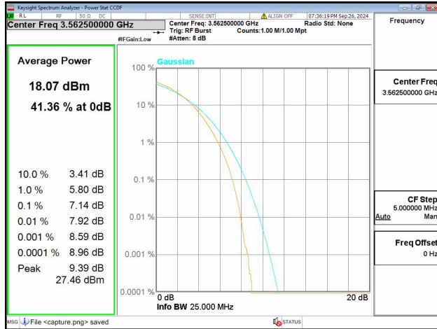
48C / 20+5MHz / Low CH / 64QAM
