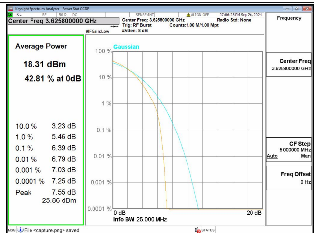
48C / 5+20MHz / Mid CH / 16QAM
