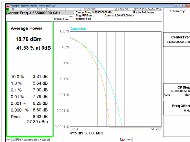
48C / 20+10MHz / Low CH / 64QAM
