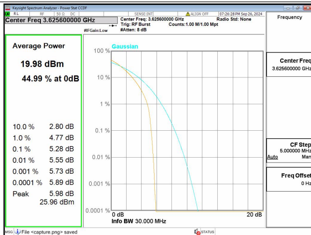
48C / 10+20MHz / Mid CH / QPSK
