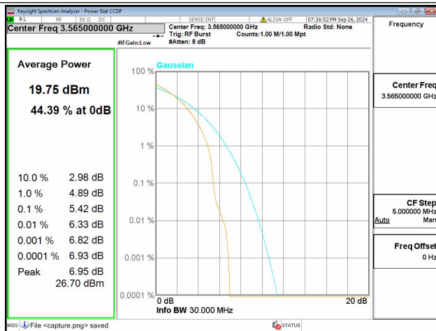
48C / 20+10MHz / Low CH / QPSK
