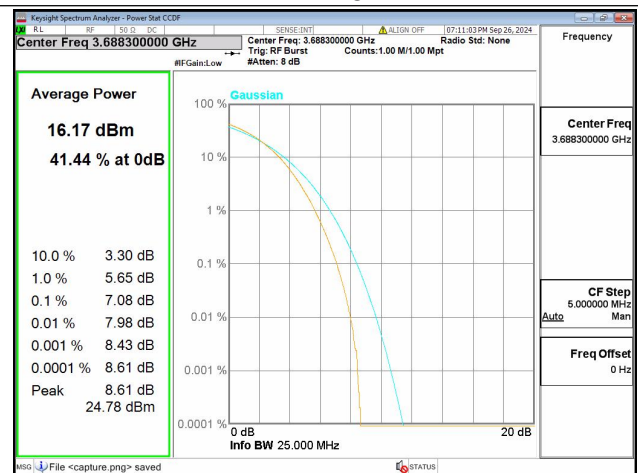
48C / 5+20MHz / High CH / 256QAM
