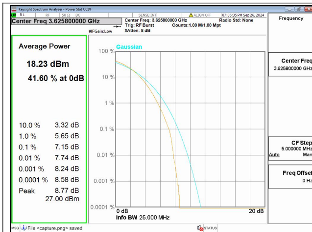
48C / 5+20MHz / Mid CH / 64QAM
