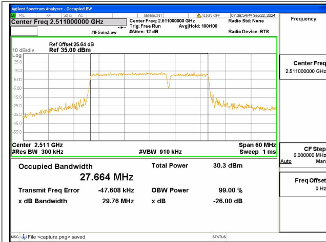
41C / 20+10MHz / 64QAM/ Low CH
