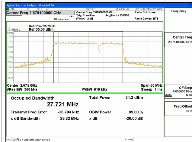
41C / 20+10MHz / QPSK/ High CH
