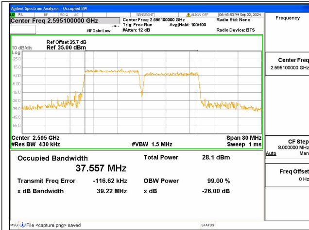
38C / 20+20MHz / 64QAM/ Mid CH
