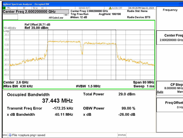
38C / 20+20MHz / QPSK/ High CH
