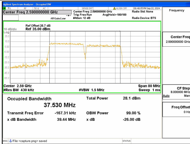
38C / 20+20MHz / 64QAM/ Low CH
