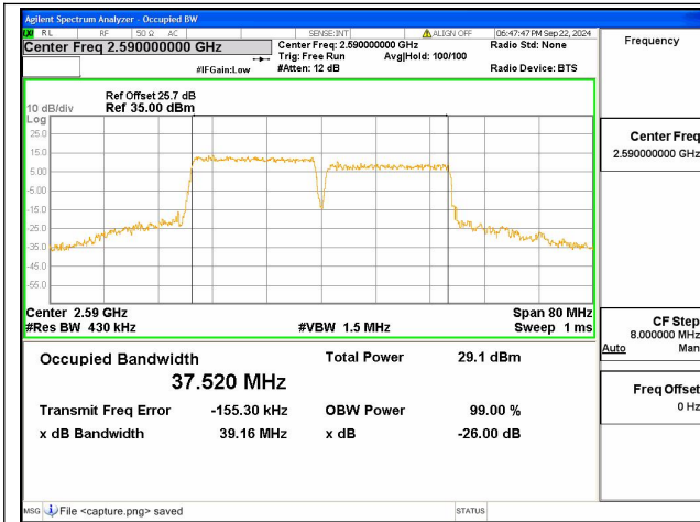
38C / 20+20MHz / QPSK/ Low CH
