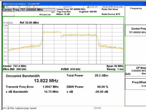
12B / 5+10MHz / QPSK/ High CH
