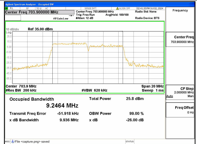
12B / 5+5MHz / 256QAM / Low CH
