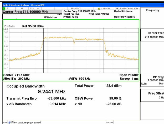
12B / 5+5MHz / QPSK/ High CH
