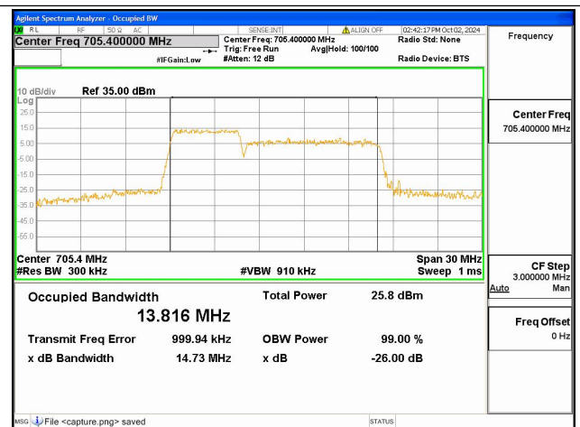
12B / 5+10MHz / 256QAM/ Low CH
