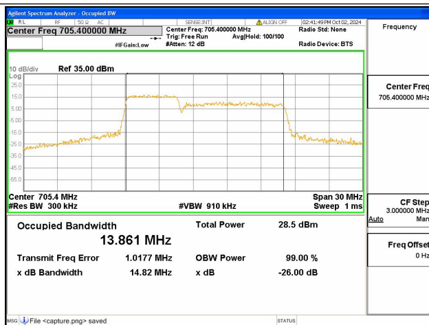
12B / 5+10MHz / QPSK / Low CH
