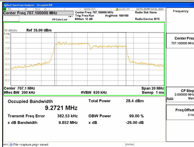
12B / 5+5MHz / QPSK/ Mid CH
