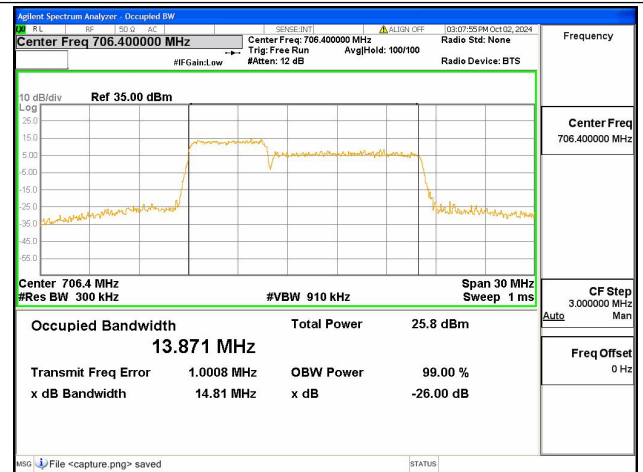
12B / 5+10MHz / 256QAM/ Mid CH
