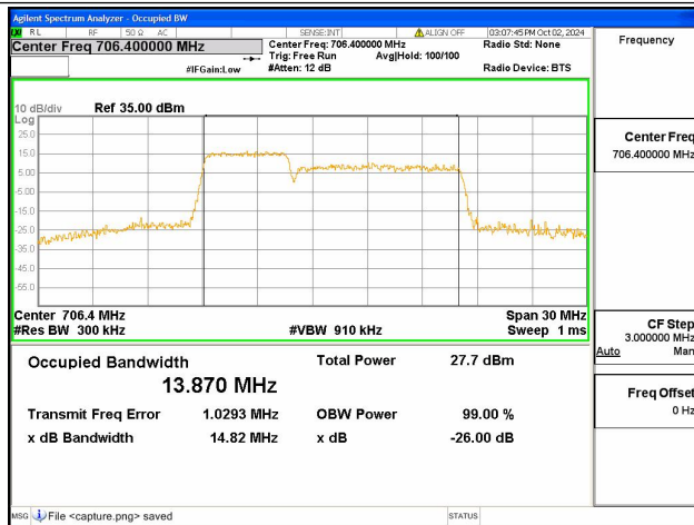
12B / 5+10MHz / 64QAM/ Mid CH
