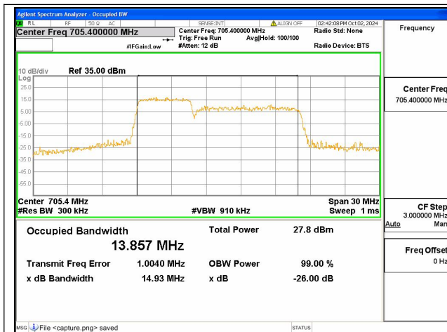
12B / 5+10MHz / 64QAM/ Low CH
