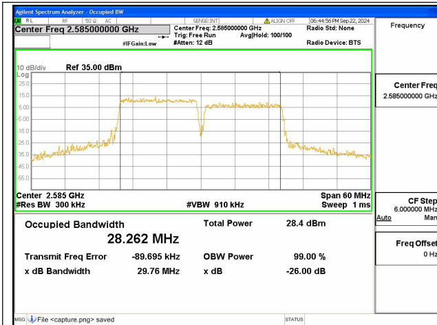
38C / 15+15MHz / QPSK/ Low CH
