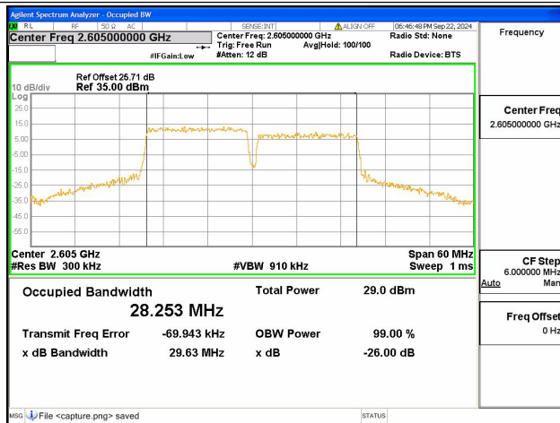
38C / 15+15MHz / QPSK/ High CH
