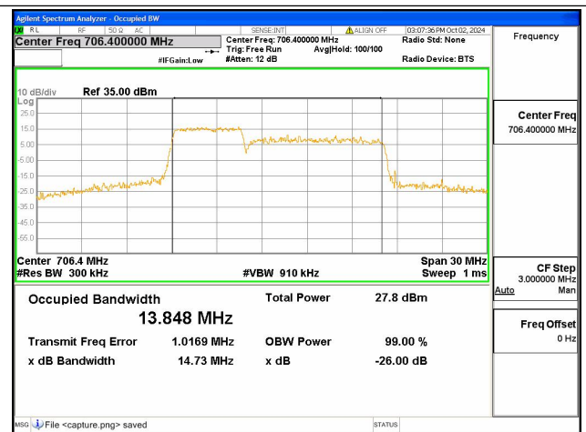
12B / 5+10MHz / 16QAM/ Mid CH
