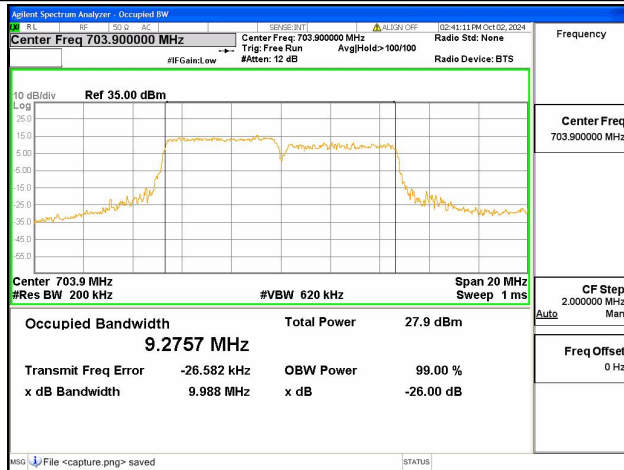
12B / 5+5MHz / 64QAM / Low CH
