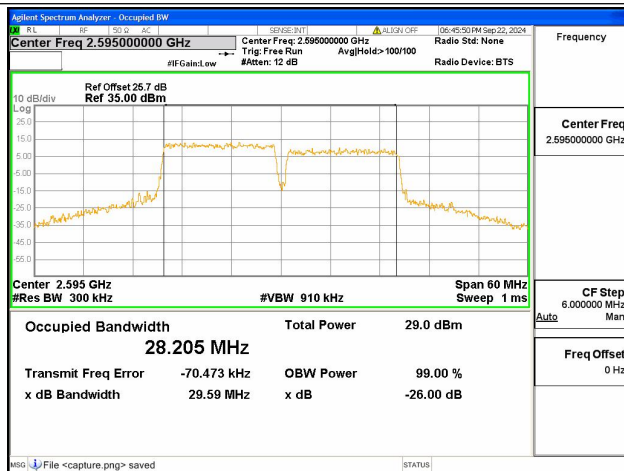
38C / 15+15MHz / QPSK/ Mid CH
