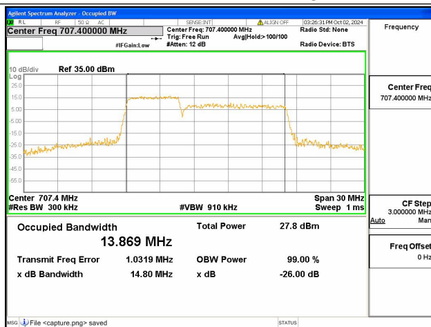
12B / 5+10MHz / 64QAM/ High CH
