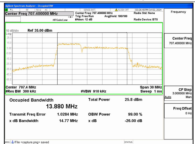
12B / 5+10MHz / 256QAM/ High CH
