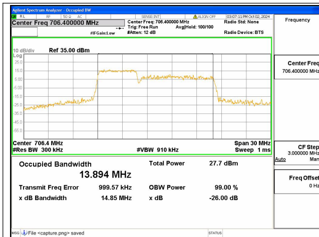
12B / 5+10MHz / QPSK/ Mid CH
