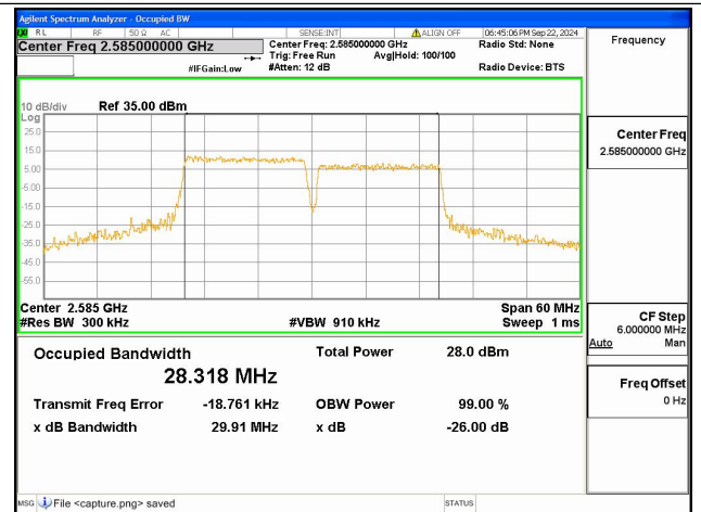
38C / 15+15MHz / 16QAM/ Low CH
