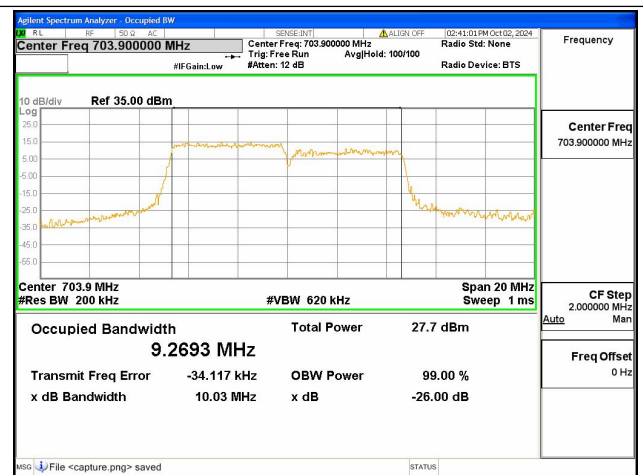
12B / 5+5MHz / 16QAM / Low CH
