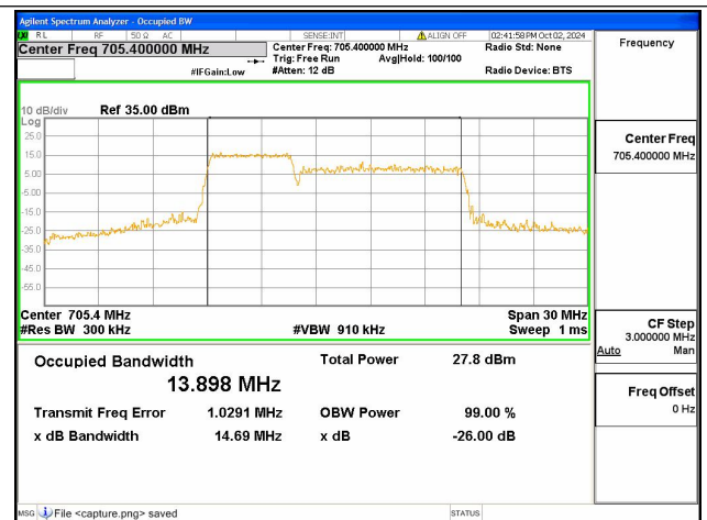
12B / 5+10MHz / 16QAM / Low CH
