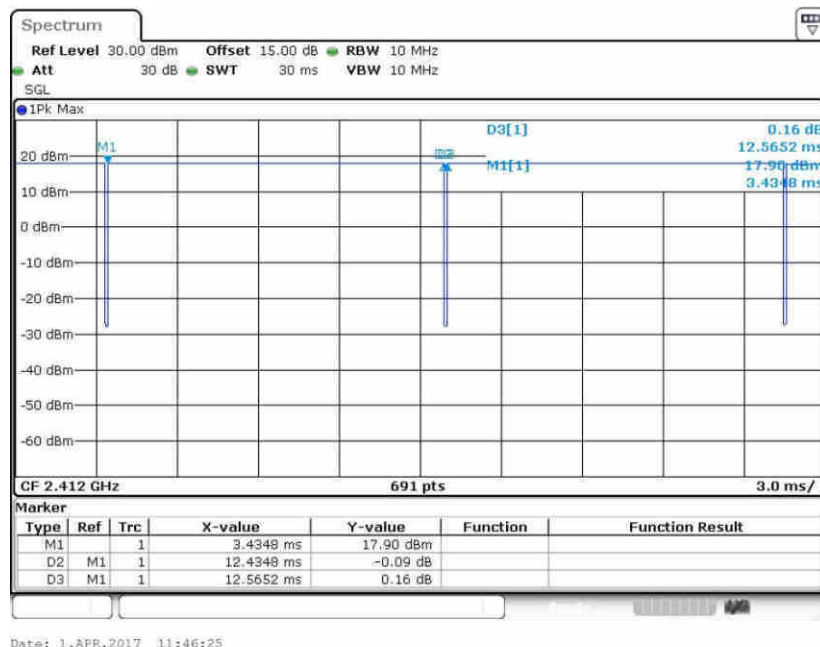
802.11b Ant.1+2
