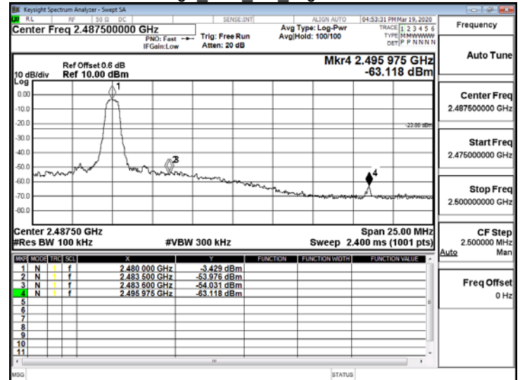
Band Edge BLE 1M HighCH39-2480
