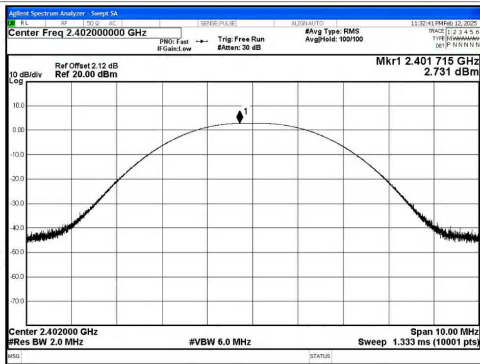
Power NVNT BLE 500Kbps 2402MHz Ant1
