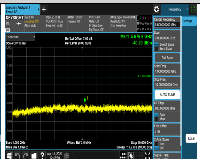
Band71-20MHz-16QAM-133222-1RB#0-Range2:1000~ 10000MHz
