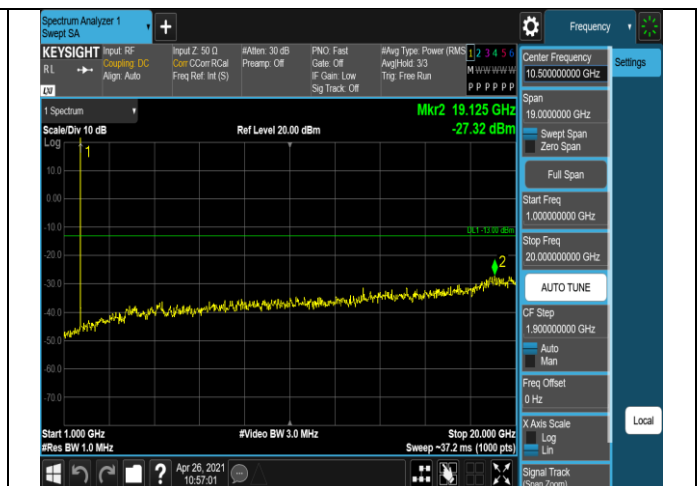
Band4-1.4MHz-QPSK-20175-1RB#0-Range2:1000~20
