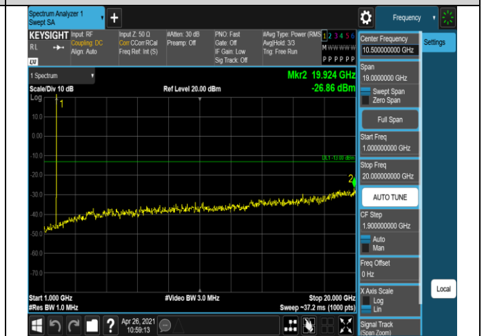
Band4-20MHz-QPSK-20050-1RB#0-Range2:1000~20000MHz
