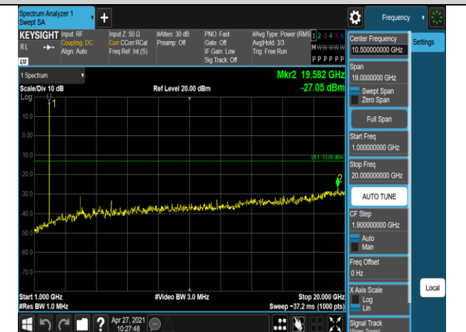
Band2-20MHz-QPSK-18700-1RB#0-Range2:1000~200
