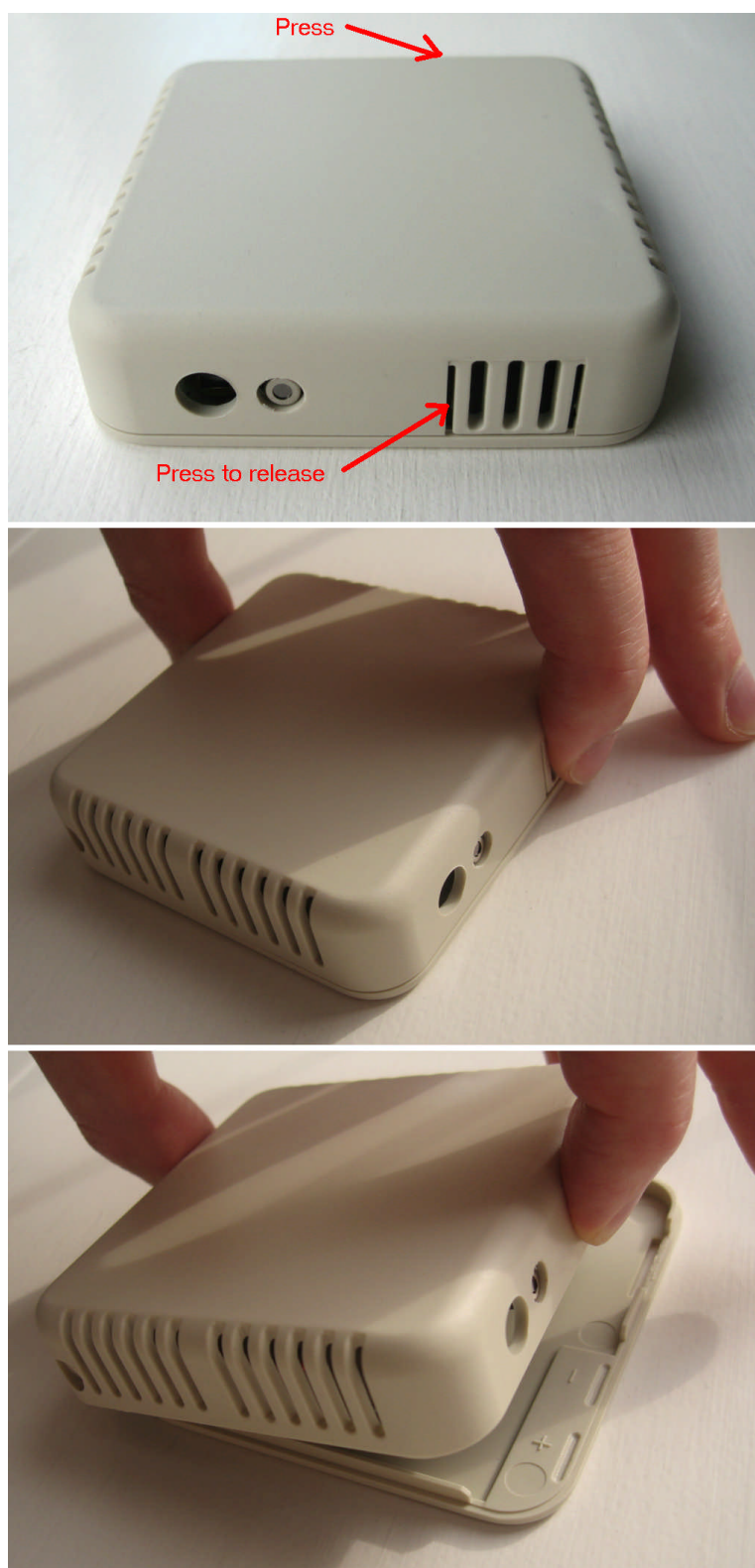
Fig. 2.0 WDC Lid Removal
